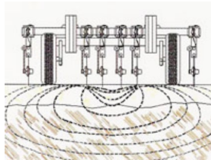
Figura 5. Un diagrama de corriente eléctrica (líneas de puntos) fluyendo entre diferentes discos en el carro de conductividad eléctrica y cómo éste es movido a través del suelo.
