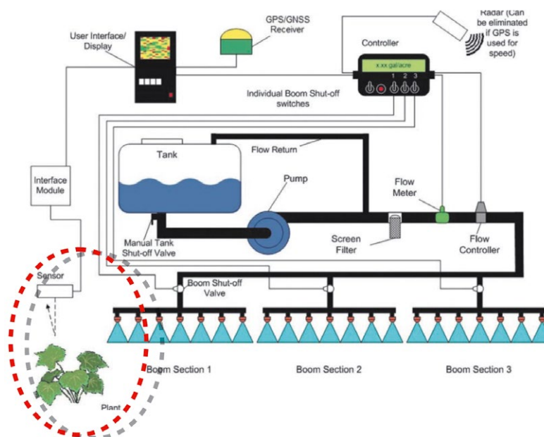
Figura 1. Esquema general del funcionamiento y los principales elementos del sistema de aplicación de dosis variable de N. En el círculo rojo se aprecia la posición del sensor en el sistema de aplicación. Fuente imagen: Taylor y Fulton (2010)
