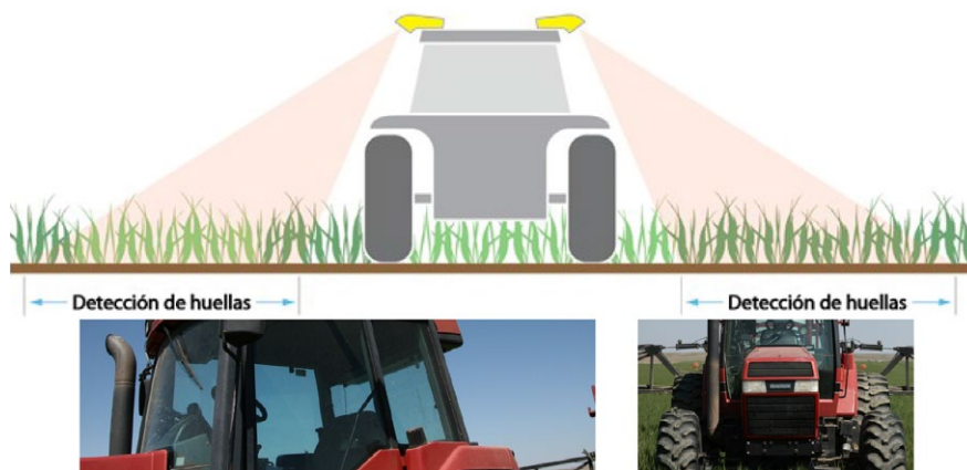
Figura 8. CropSpecTM de Topcon (a) el sensor va montado en el techo del tractor para el sensoramiento de los índices vegetacionales. Este sensor mide en forma oblicua a medida que se realiza el escaneo y la aplicación en tiempo real en el campo. Fuente imagen: Topcon
