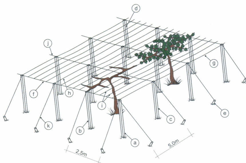
Figura 1. Sistema de condução da videira em latada, especificando postes e fios. Postes: a) cantoneira; b) cabeceira; c) lateral; d) interno; e) rabicho; Fios: f) cordão primário de cabeceira; g) cordão primário lateral; h) fio da produção; i) fio da vegetação; j) fio de sustentação da malha; k) fio rabicho. (Ilustração: Alberto Miele e Luciana Prado).
