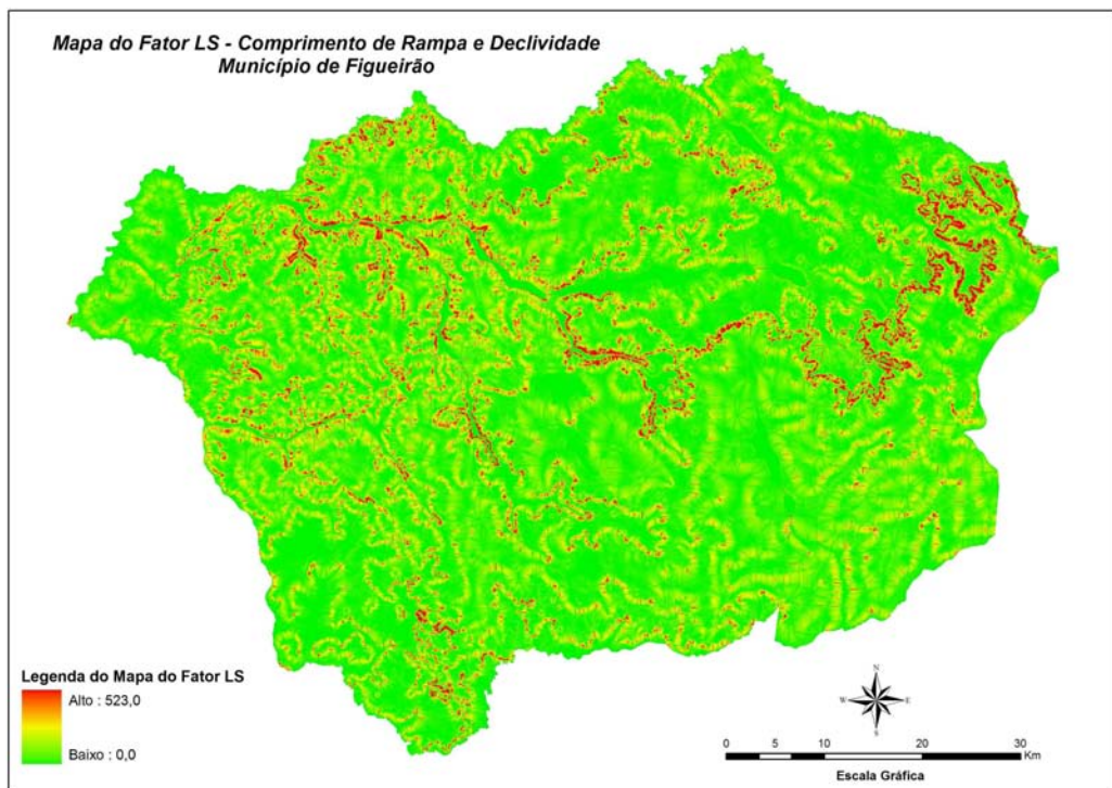
Figura 5. Mapa do fator topográfico – LS do município de Figueirão, MS.
