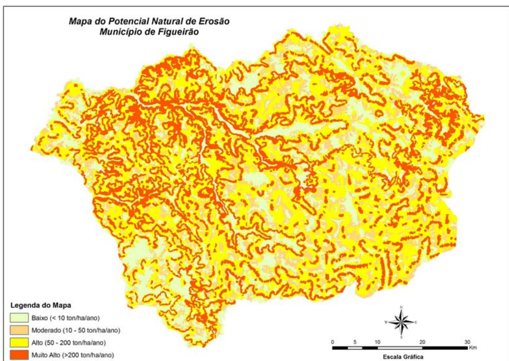
Figura 6. Mapa de classes do Potencial Natural de Erosão (PNE) do município de Figueirão, MS.
