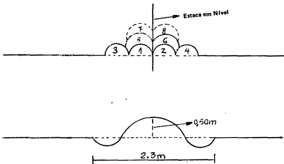
FIGURA 3 — Terraço de Base Estreita tipo MANGHUM
