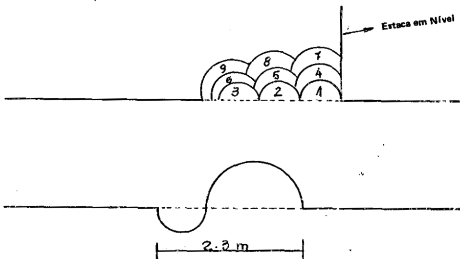
FIGURA 2 — Terraço de Base Estreita tipo NICHOLS
