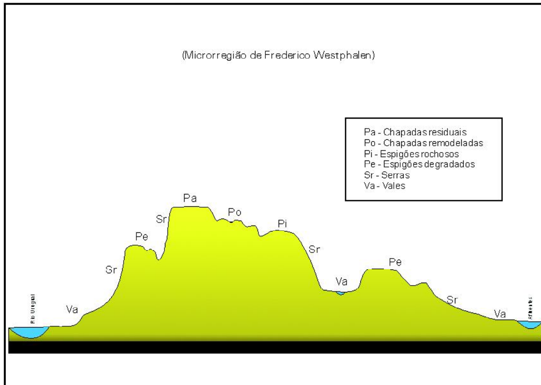
Figura 18, seção transversal do relevo de municípios do Alto Uruguai RS. Henrique da Silva Couto
