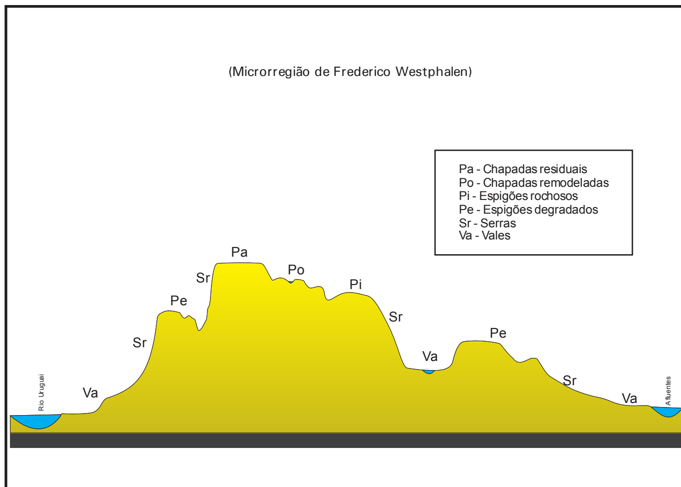
Fig 23: Secção transversal do relevo de municípios do Alto Uruguai, RS
