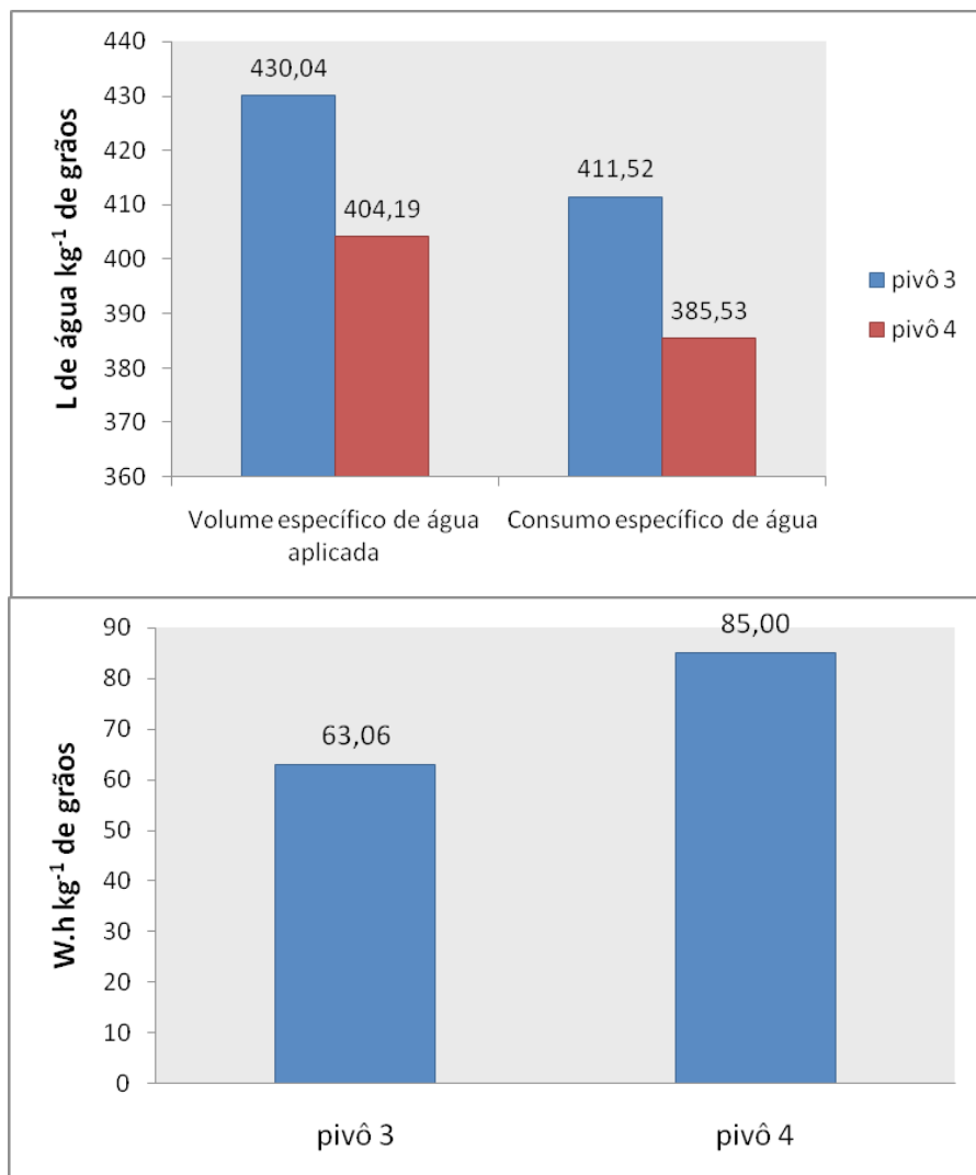
Figura 1. Acima: Volume bruto específico de água aplicada e consumo específico de água (em litros de água kg -1 de grãos produzidos) nos pivôs 3 e 4. Abaixo: Consumo específico de energia elétrica (em W.h kg -1 de grãos produzidos) para bombeamento de água nos pivôs 3 e 4 da Fazenda Guaicuí - Várzea da Palma (Fonte: ALBUQUERQUE et al., 2010)
