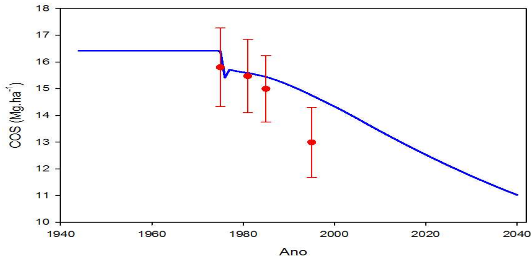
Figura 2. Simulação do carbono orgânico do solo (linha) e valores observados (pontos) em fazenda do Pantanal Sul-Mato-Grossense.
