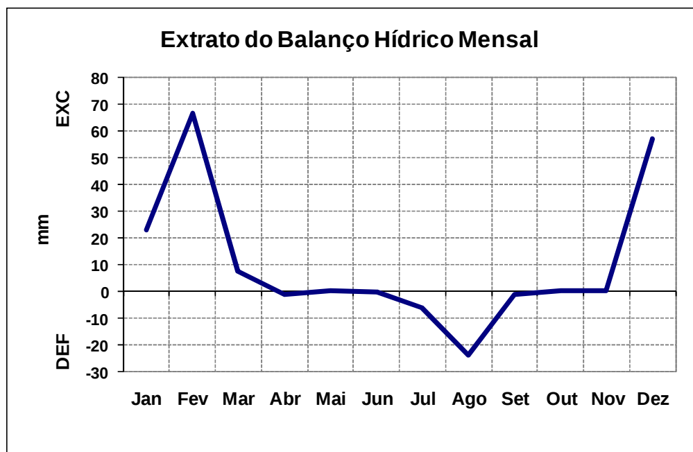
Figura 2. Representação gráfica do balanço hídrico para o município de Rochedo, Estado do Mato Grosso do Sul.
