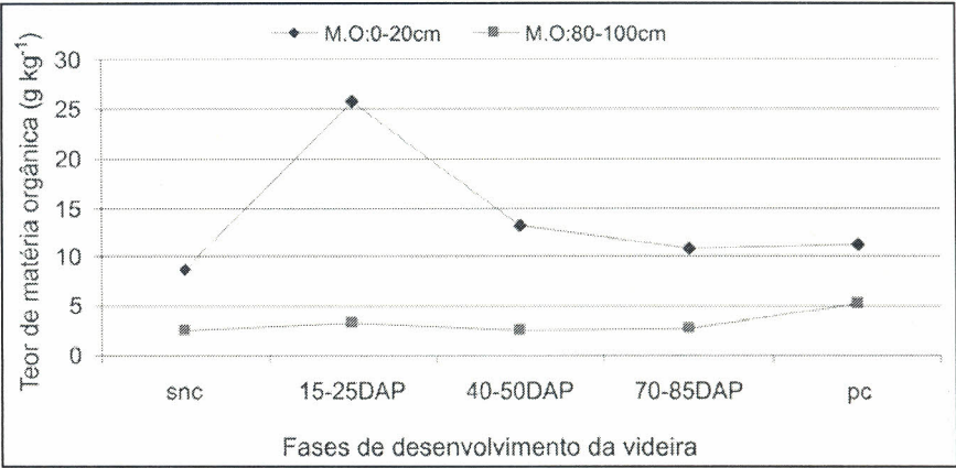
Figura 4. Teores de matéria orgânica (MO) no solo não cultivado (S NAT ) e nos lisímetros com videira aos 15-25 dias após a poda (DAP), 40-50 DAP, 70-85 DAP e no período de chuvas, após a colheita (Pchuvoso).
