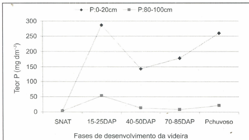
Figura 3. Teores de fósforo (P) no solo não cultivado (SNAT) e nos lisímetros aos 15-25 dias após a poda (DAP), 40-50 DAP, 70-85 DAP e no período de chuvas (Pchuvoso), após a colheita.
