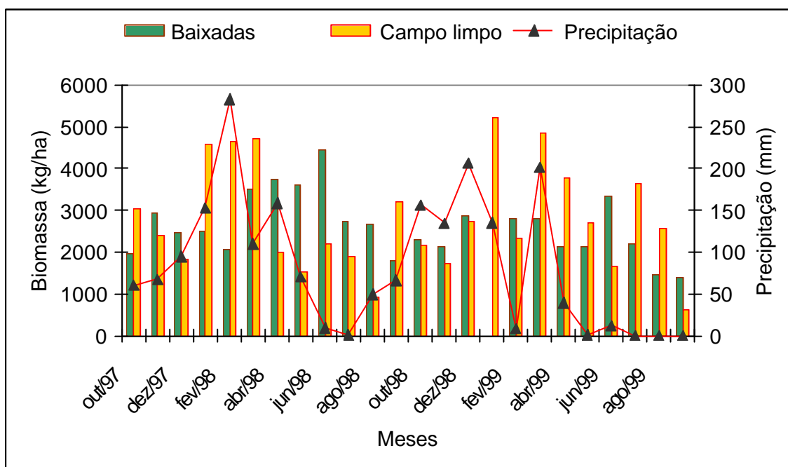
Fig. 1. Valores de disponibilidade de biomassa (Kg/ha) das fitofisionomias de campo limpo e baixadas, precipitação pluvial (mm), no período de out/97 a nov/99, fazenda Nhumirim, Pantanal, MS.
