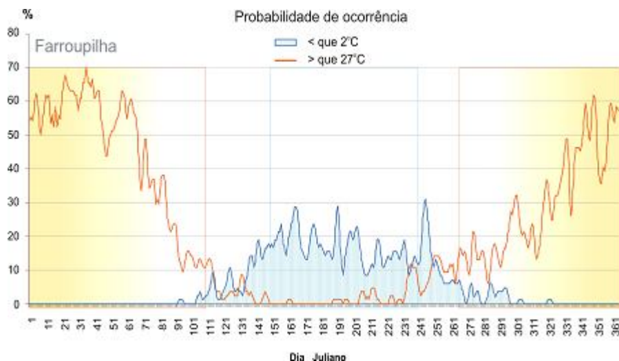
Figura 3. Frequência da temperatura máxima (superior a 27°C) e mínima absoluta (inferior a 2°C) em Farroupilha – RS. Org.: Ivan Rodrigues de Almeida.
