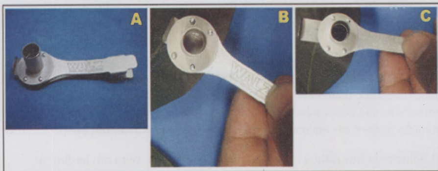
Fig. 1. A) Clipe de escurecimento foliar do fluorômetro PAM-2000 (Heinz Walz, Alemanha). B) Clipe fechado escurecendo uma área de cerca de 0,38 cm 2 . C) Clipe aberto após a medição da fluorescência. O clipe deve ser aberto somente após a introdução da fibra óptica para a medição da fluorescência.
