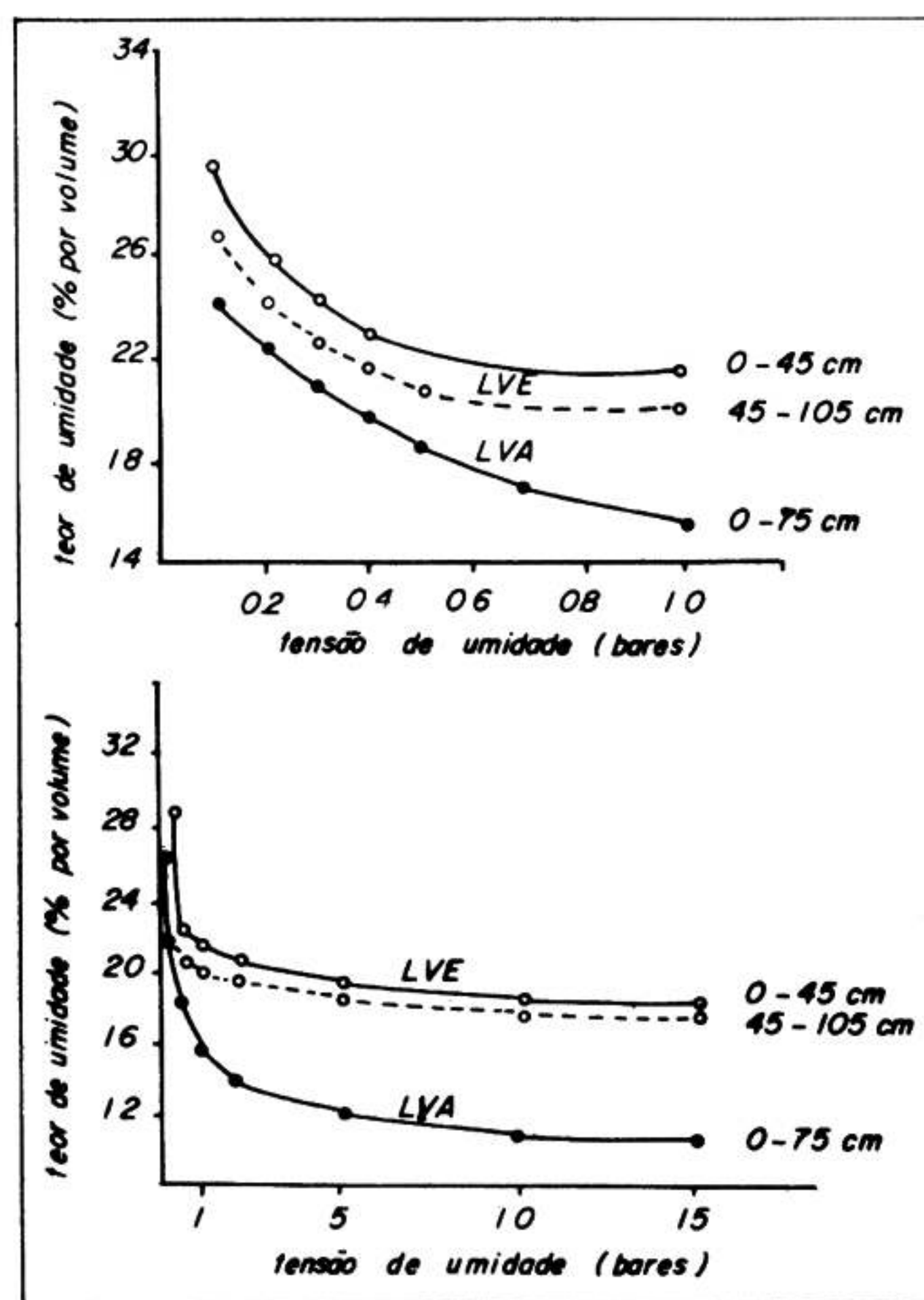
FIGURA 40. Curvas de tensão de umidade do solo (0-1 e 0-15 bars) para os solos LVE e LVA.
