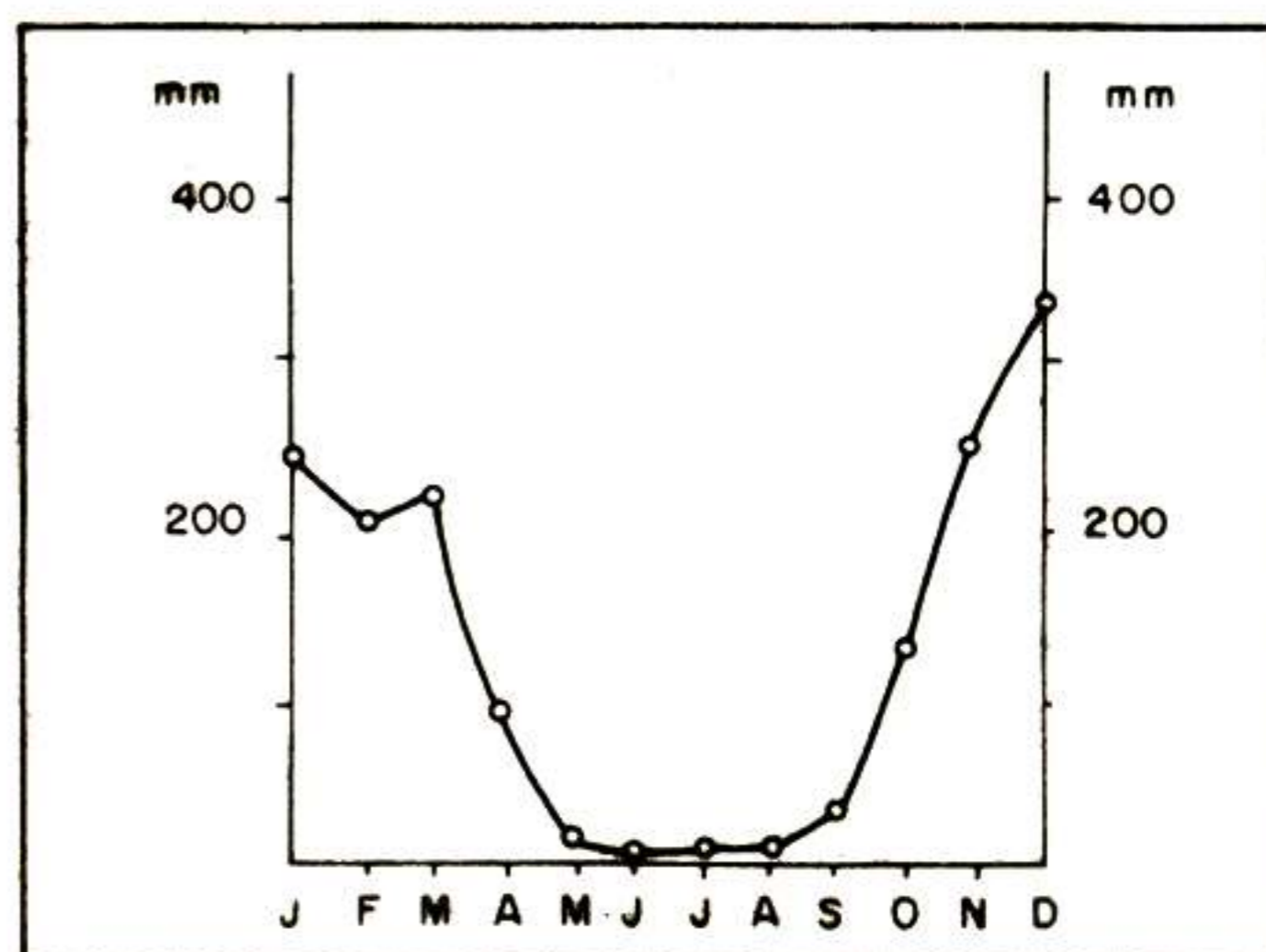
FIGURA 2. Precipitação típica da área dos Cerrados — média de 40 anos — Formosa — Goiás
