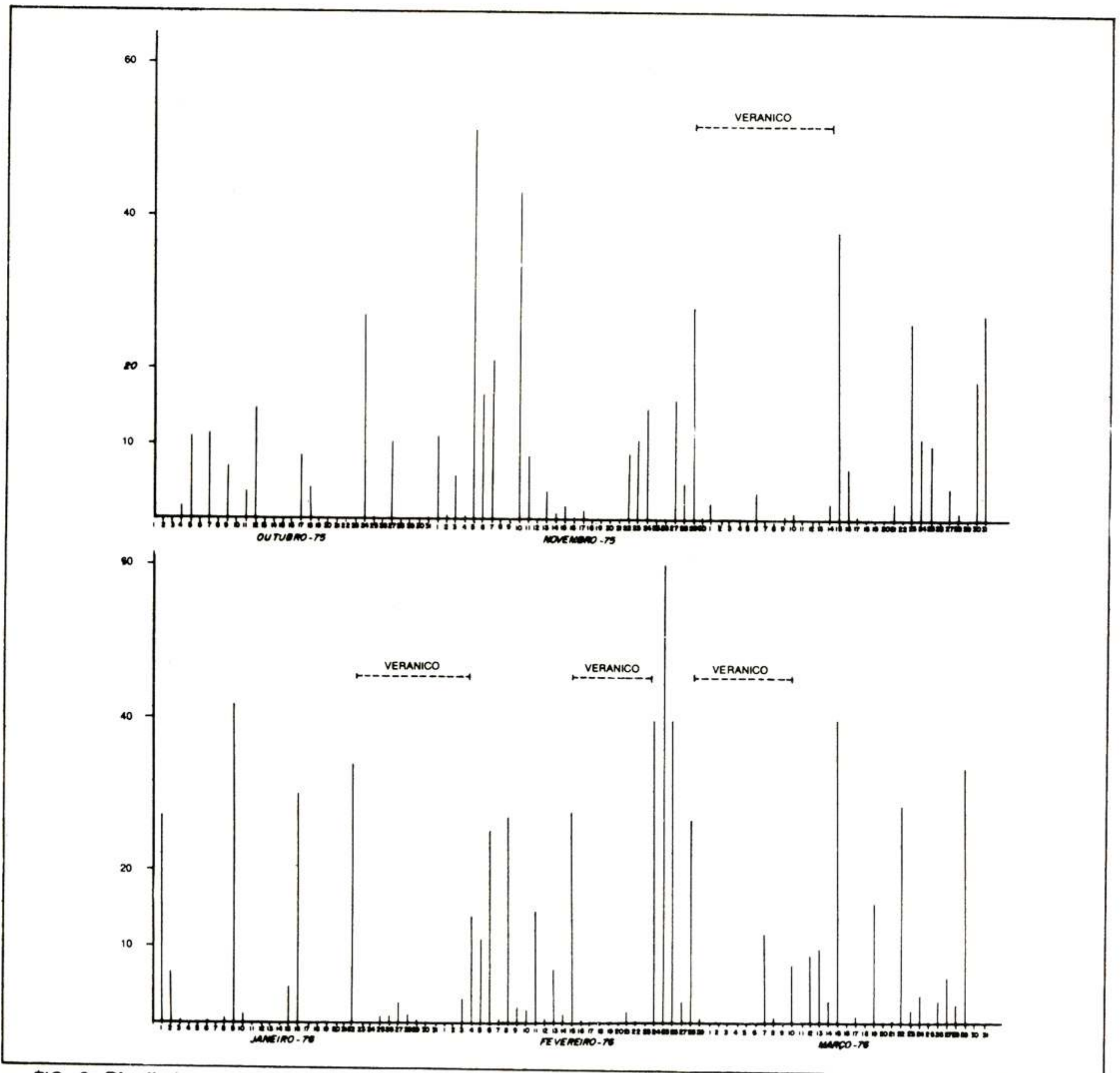
FIG 3. Distribuição diária da precipitação pluviométrica, na época das chuvas, no ano agrícola 1975-1976, na sede do CPAC.
