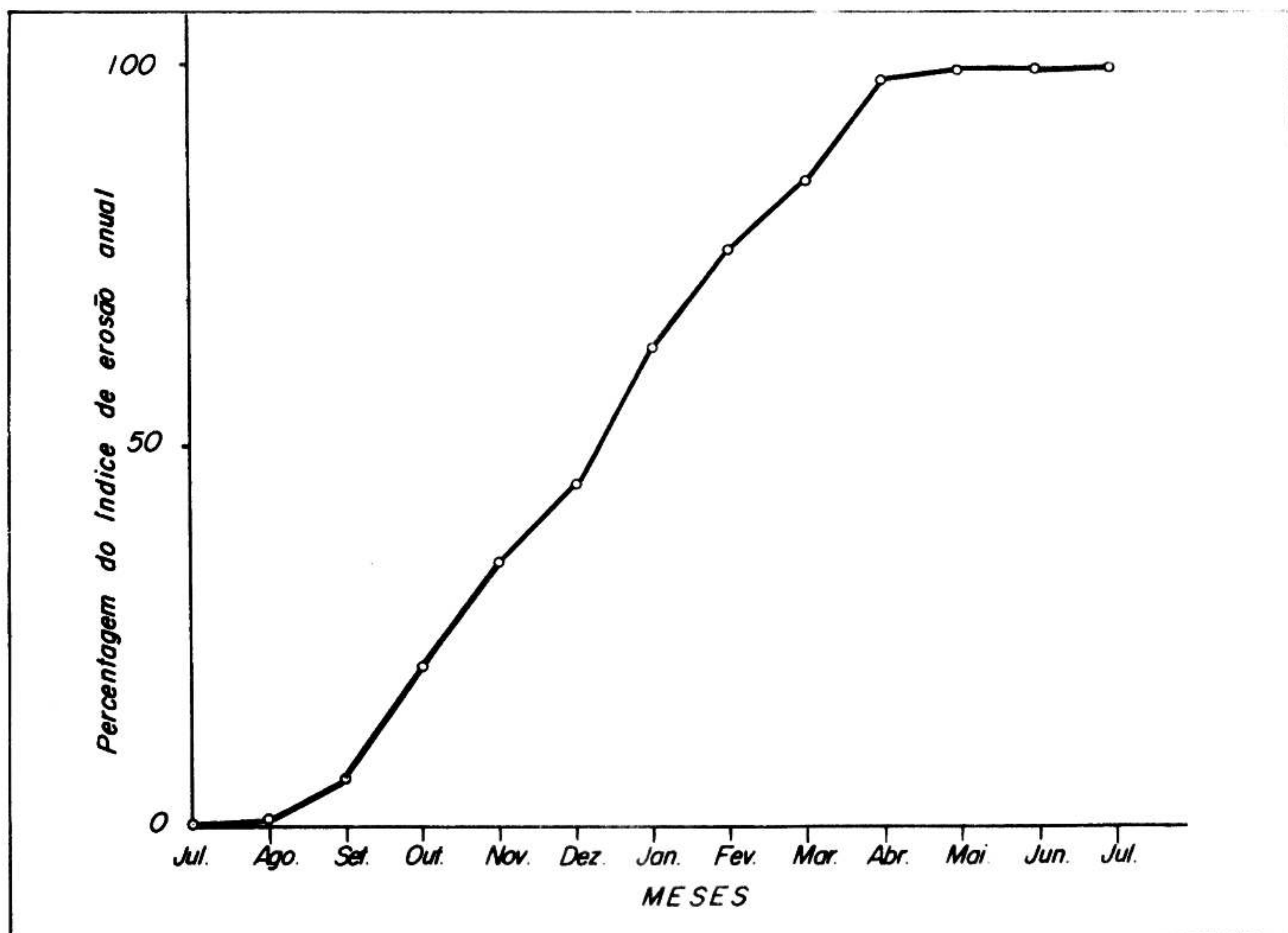
FIG 42. Distribuição anual do índice de erosão acumulado. UEPAE/BRASÍLIA, 1970/76.
