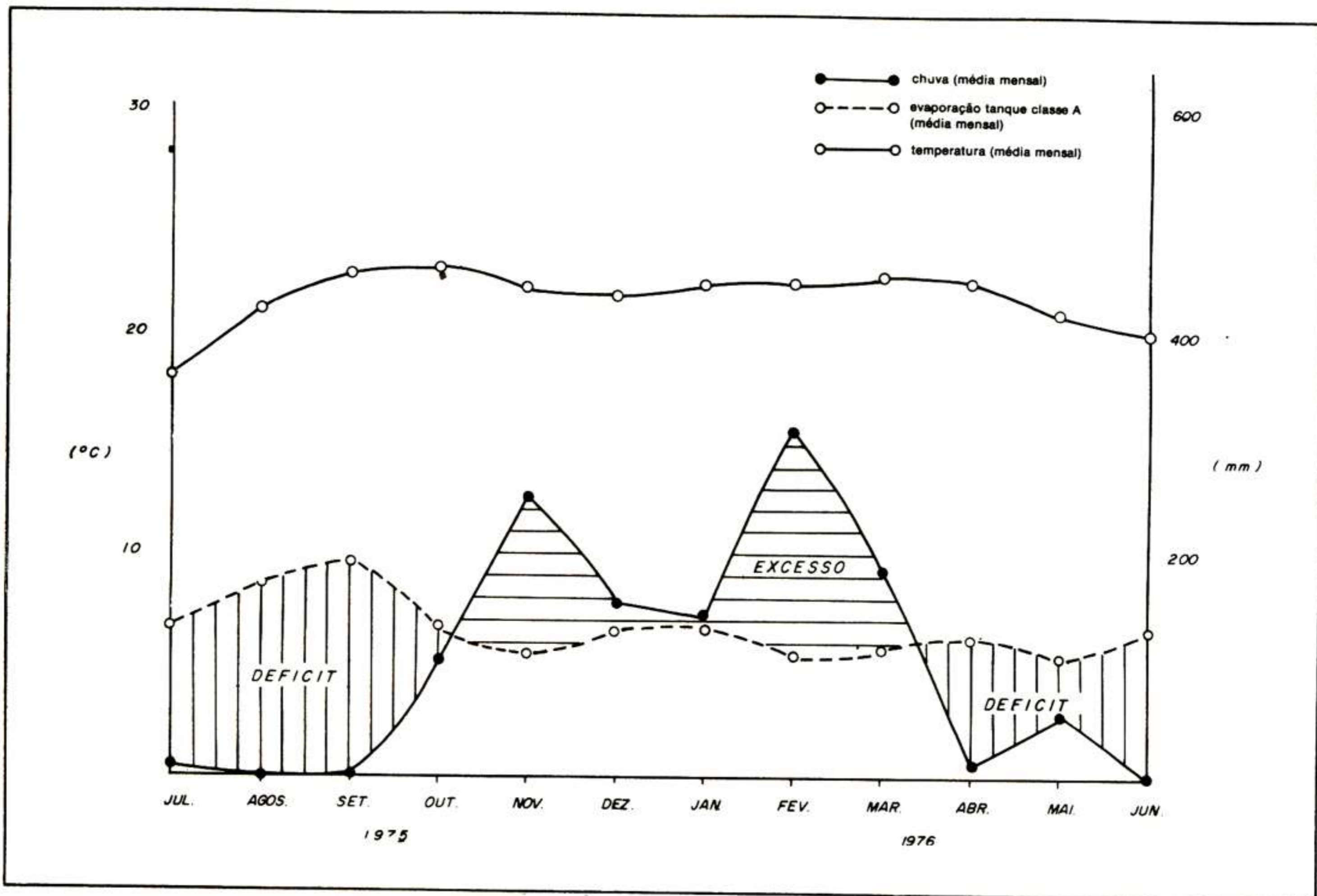
FIGURA 5. Balanço hídrico e temperatura média mensal, no CPAC, durante o ano agrícola julho-1975 a junho-1976.
