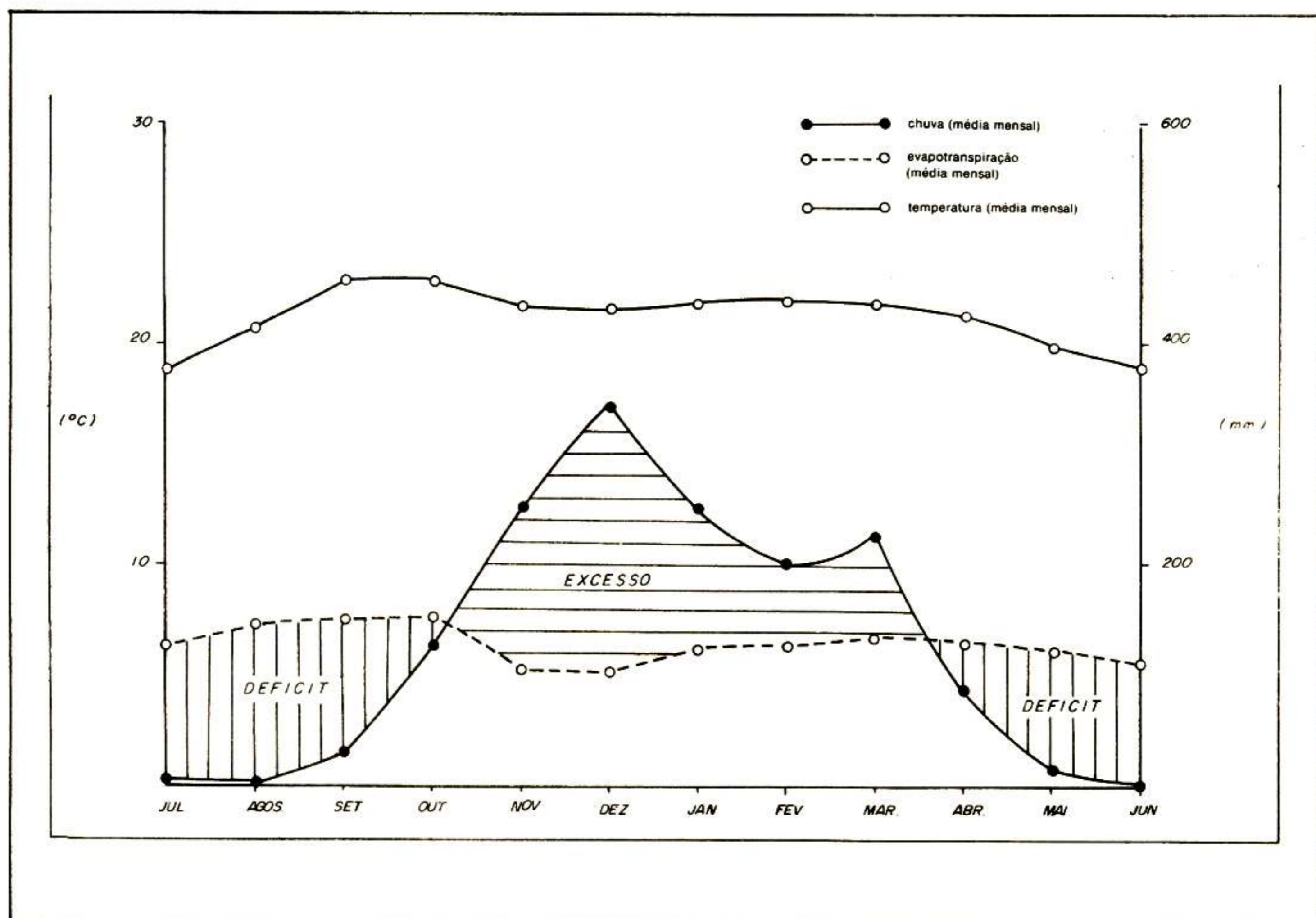
FIGURA 4. Balanço hídrico e temperatura média mensal de 35 anos de observações, em Formosa-Go, calculado segundo Hargreaves.
