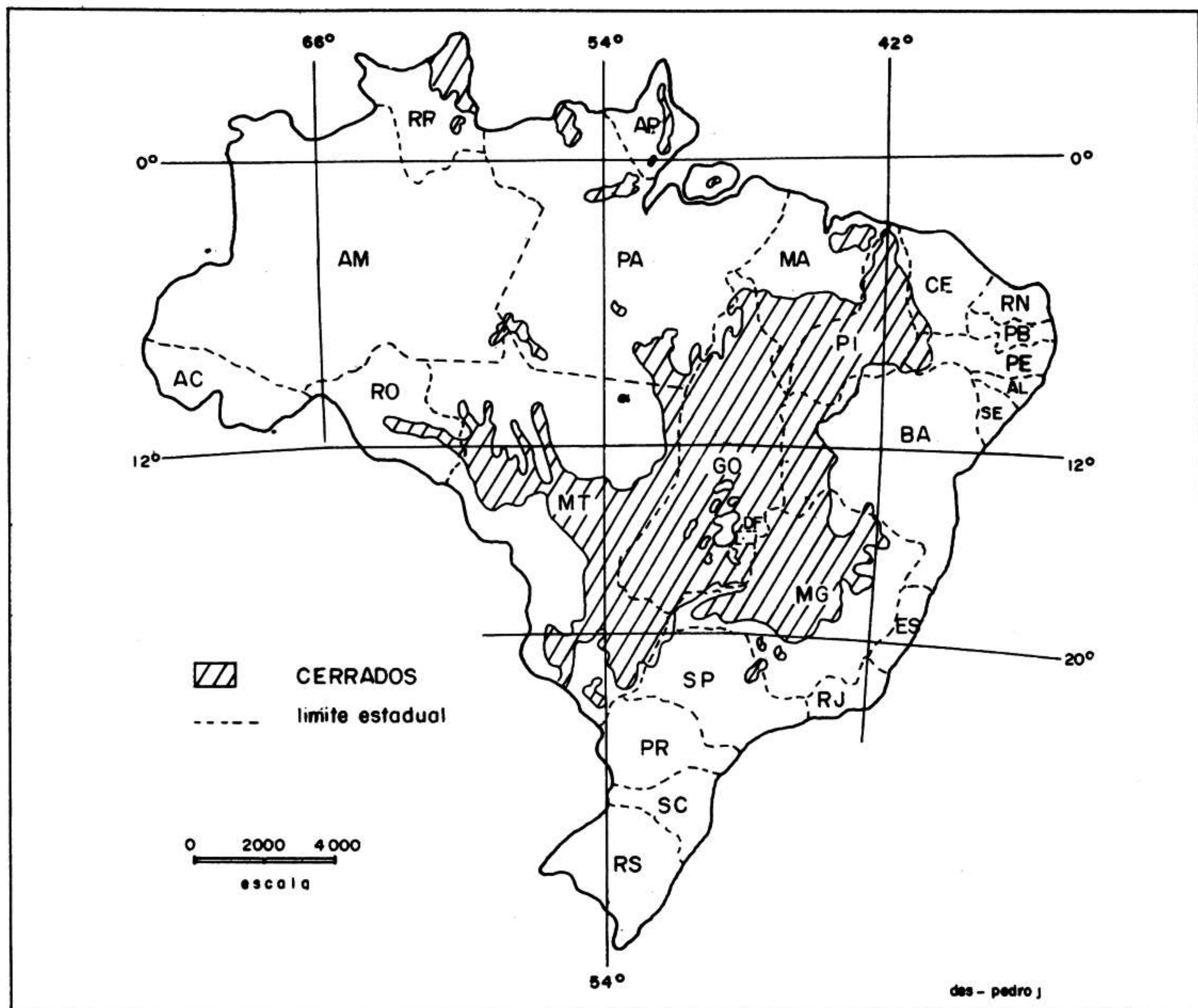
FIGURA 1. Estádio atual do conhecimento sobre a distribuição dos Cerrados, incluídas as áreas de transição com outras formações.
