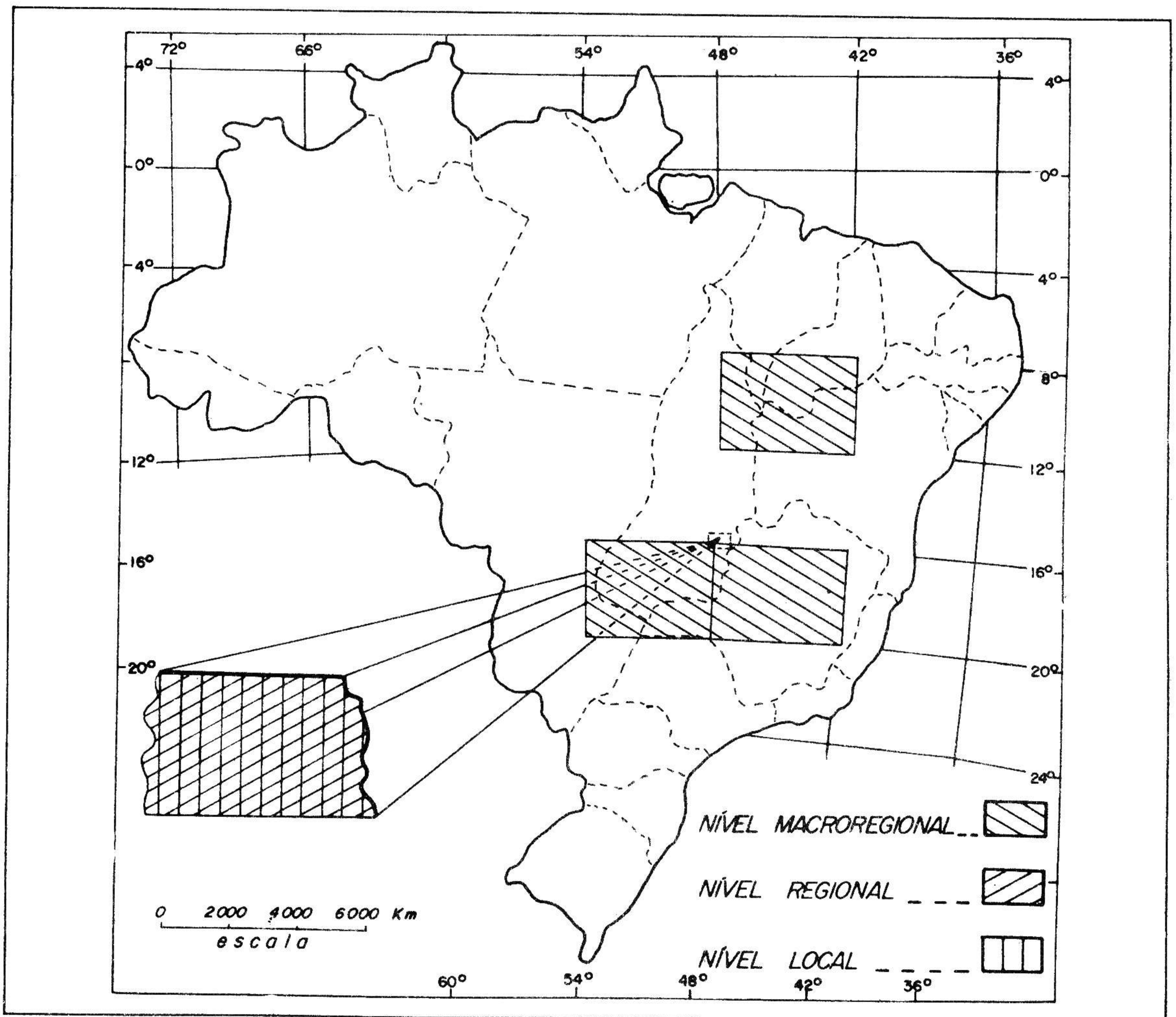
FIG. 8. Áreas Prioritárias de Atuação do Projeto Inventário.
