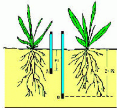
Figura 3. Profundidades de instalação dos tensiômetros, mostrando a localização do tensiômetro de controle da irrigação (ponto A – profundidade P1) e o do controle do excesso ou déficit de irrigação (ponto B – profundidade P2 = profundidade efetiva do sistema radicular Z).
