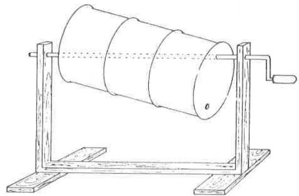
Fig. 2. Tambor giratório com eixo excêntrico para tratar sementes (Desenho: Danilo Estevão).
