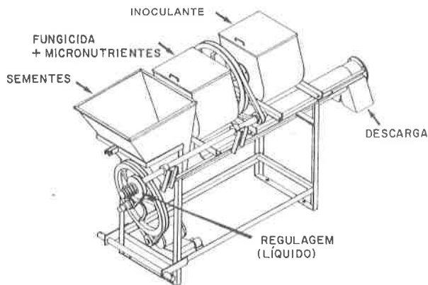
Fig.1. Máquina de tratar sementes (Adaptado de Grazmec).
