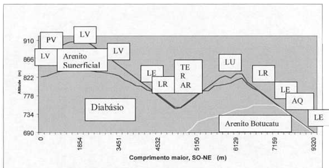
Figura 8 - Perfil topográfico ao longo do eixo mais longo (SO-NE), geologia e distribuição de solos na fazenda Cachim.
