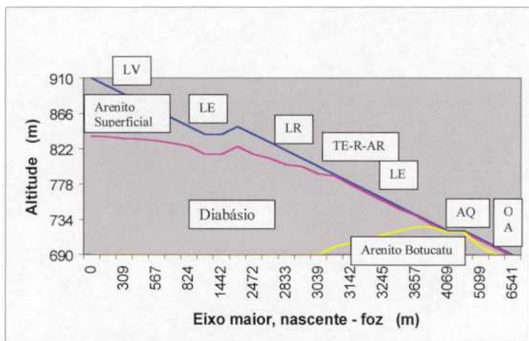
Figura 9 - Perfil topográfico ao longo do eixo mais longo (nascente-foz), geologia e distribuição de solos, na microbacia hidrográfica do ribeirão Cachim.
