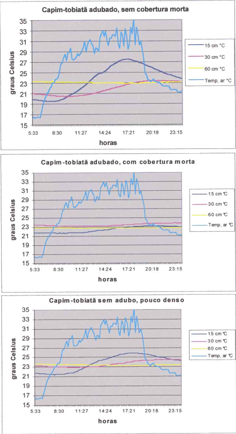
Figura 3. Variação da temperatura em um Latossolo Vermelho-Amarelo, na fazenda Cachim, ocupado por vegetação de capim-tobiatã ( Panicum maximum ), com diferentes graus de cobertura de solo, em 20/11/1997. Fonte: André Torres (1997) (Embrapa Instrumentação Agropecuária; não publicado)
