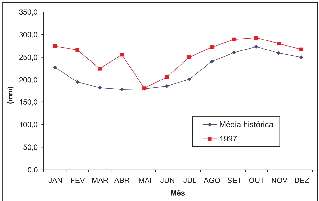
FIG. 4. Evaporação do tanque “Classe A”, totais mensais e anual em Paraibapa, 1997, comparada com a média histórica (1975-1997).
