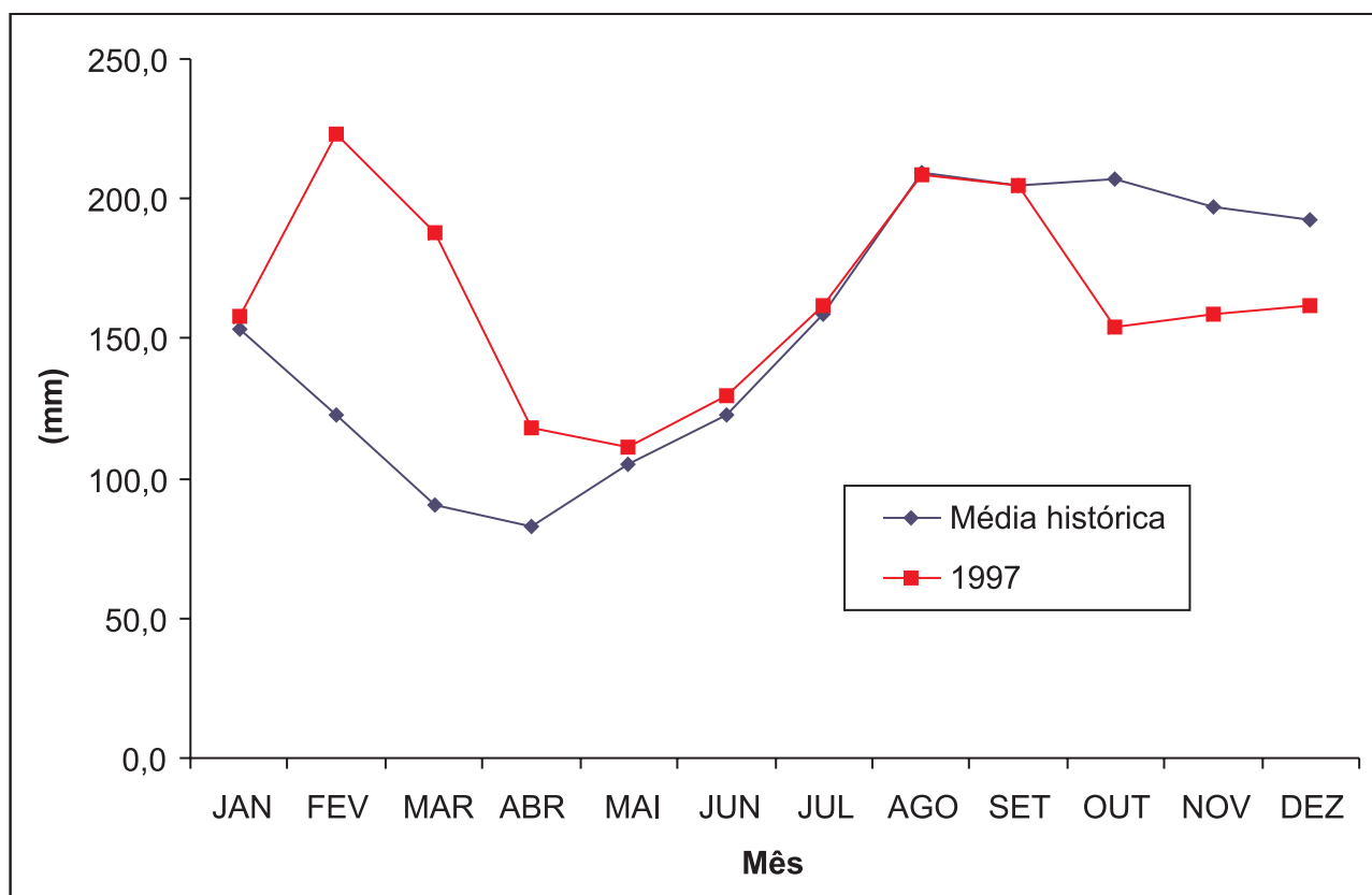
FIG. 5. Evaporação de Piche, totais mensais e anual em Paraipaba,1997, comparada com a média histórica (1975-1997).
