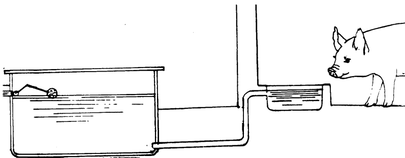
FIG. 9. Bebedouro com sistema de bóia.
