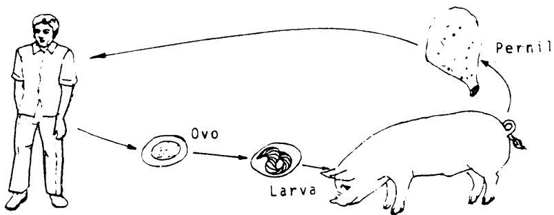
FIG. 14. Ciclo da cisticercose.
