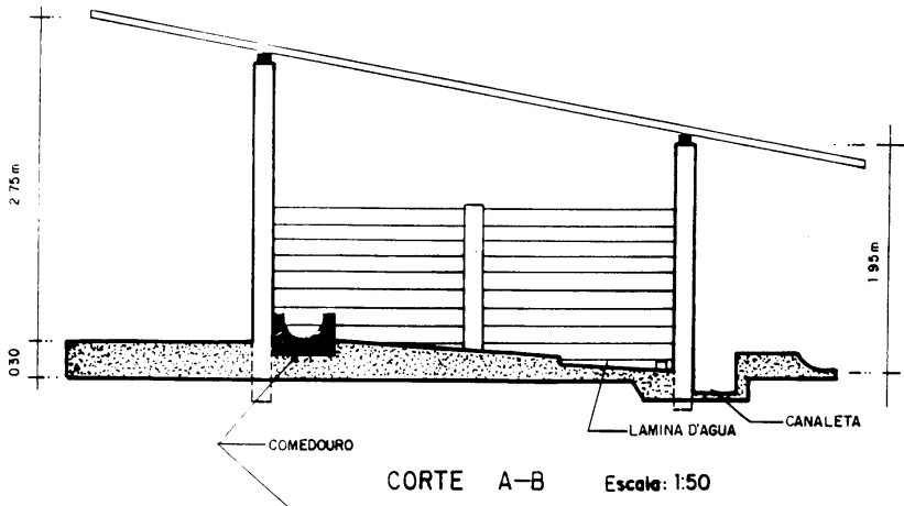
FIG. 5. Vista da instalação com detalhes.
