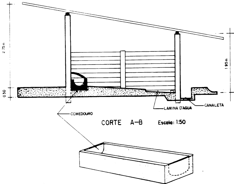
FIG. 6. Comedouro de suínos construído de alvenaria.
