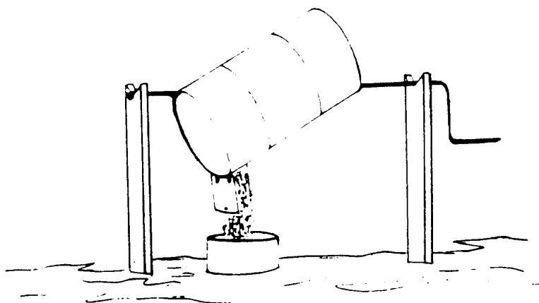
FIG. 10. Misturador de tambor.
