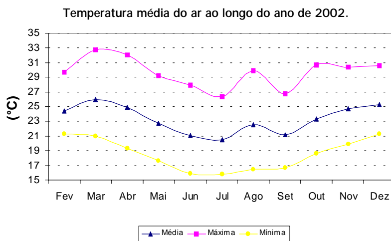
Fig. 2 - Variação da temperatura do ar ao longo do ano de 2002.
