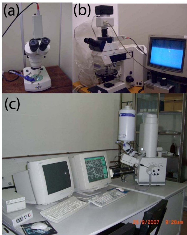
Fig. 1. Equipamentos de microscopia utilizados: (a) Lupa; (b) Microscópio Ótico com Luz Polarizada; (c) © FEG-MEV.
