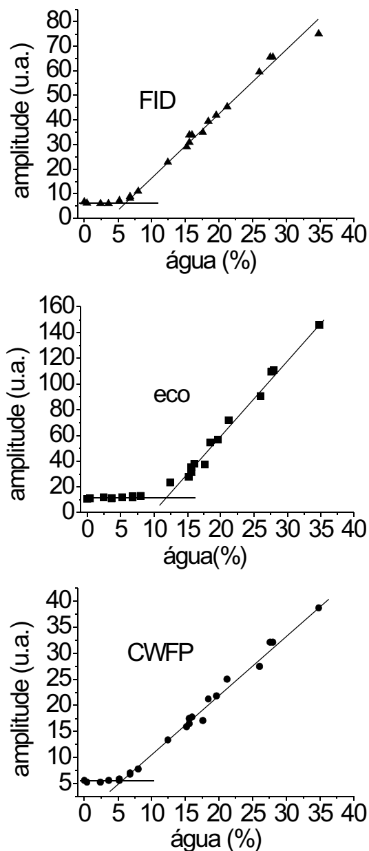
Figura 4. Medidas da amplitude dos sinais de RMN, FID (A), Eco (B) e CWFP (C) para sementes de trigo com diferente umidade.
