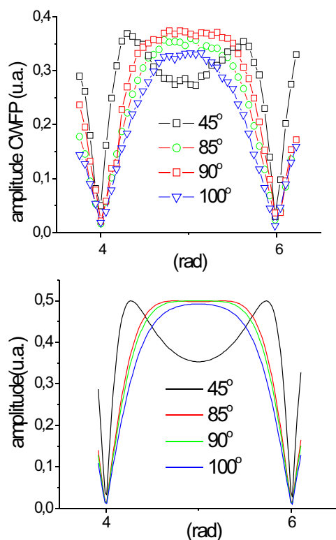
Figura 1. Variação da amplitude do sinal CWFP em função de \alpha ( 45, 80, 90 e 100 graus) e \alpha ( 3,8 a 6,2 ). A) Experimental e B) Calculado pela equação 1.
