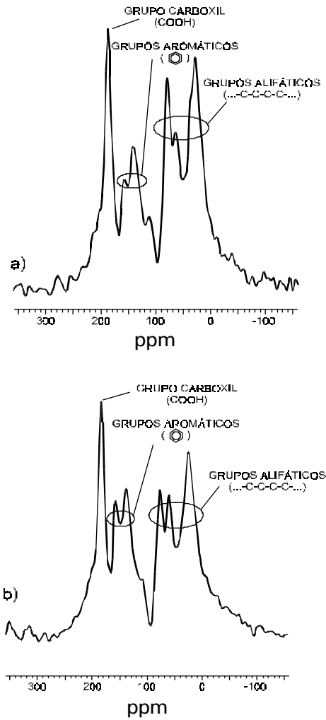
Figura 1 - Espectros de RMN 13C de ácidos húmicos da camada superficial (0-5cm) de um latossolo roxo, sob os seguintes manejos: a) manejo convencional; b) plantio direto.
