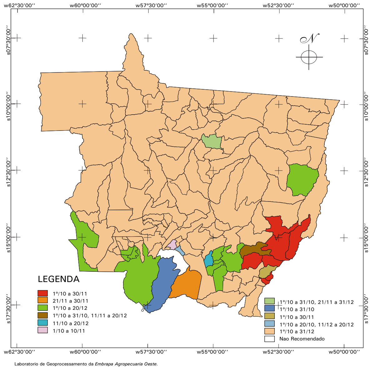
FIG. 1. Épocas de semeadura para a cultura da soja de ciclos semitardio e tardio, em solos de média baixa capacidade de armazenamento de água, no Estado de Mato Grosso.
