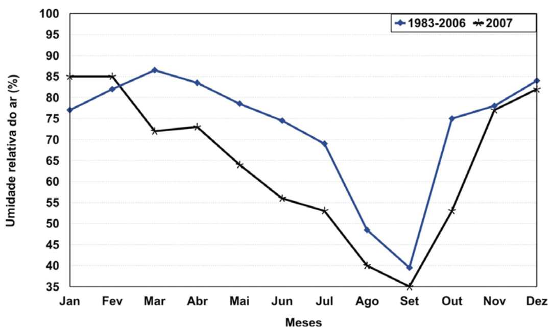
Fig. 4. Umidade relativa do ar (1983-2006 e dados de 2007), médias mensais, do município de Santo Antônio de Goiás-GO.
