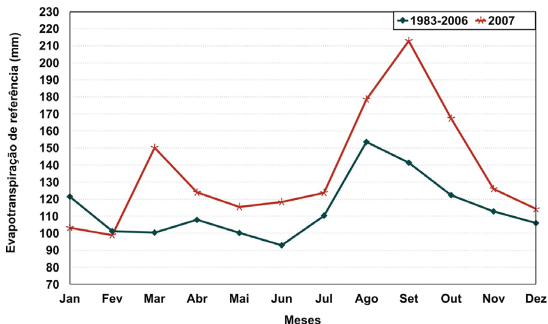
Fig. 3. Evapotranspiração de referência (1983-2006 e dados de 2007), estimada pelo método de Penman-Monteith, médias mensais, do município de Santo Antônio de Goiás-GO.
