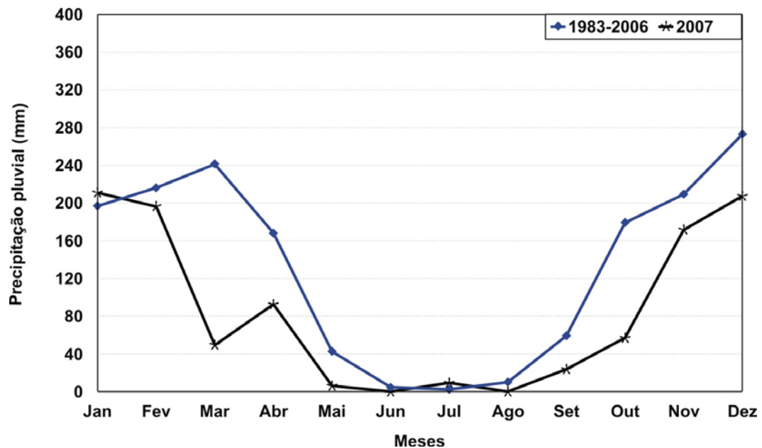
Fig. 2. Precipitação pluvial (1983-2006 e dados de 2007), médias mensais, do município de Santo Antônio de Goiás-GO.
