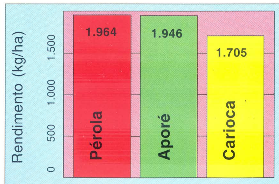
FIG. 1. Rendimento (kg/ha) das cultivares Pérola, Aporé e Carioca, em Goiás e no Distrito Federal. Média de 20 ensaios.
