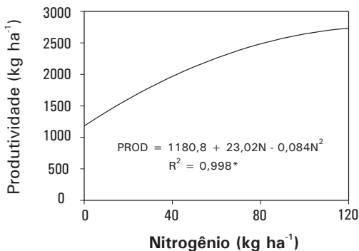
FIG. 2. Produtividade do feijoeiro, cultivar Aporé, em resposta às doses de nitrogênio aplicadas em cobertura (médias de 1997 e 1998).
