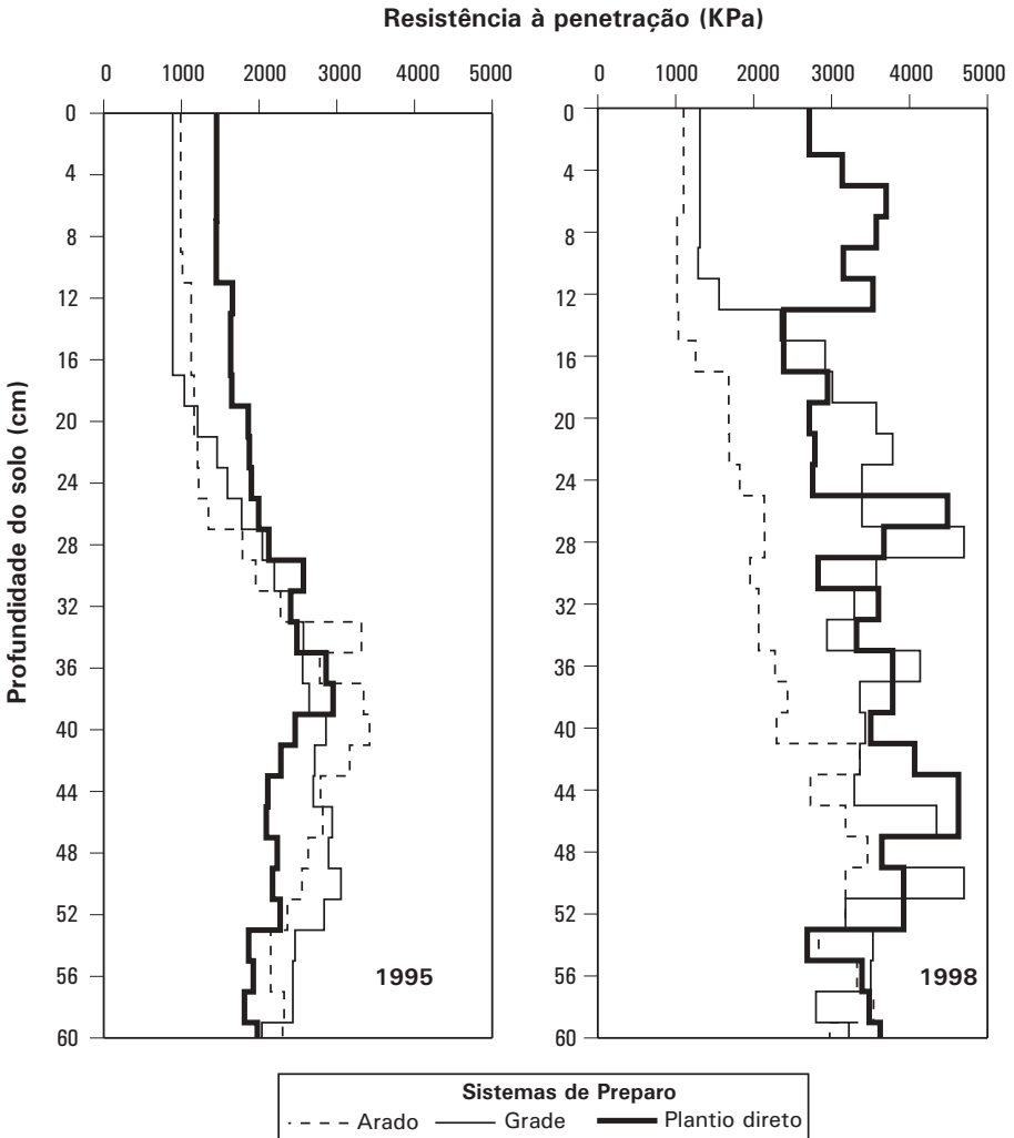
FIG. 1. Resistência do solo à penetração, no perfil de 0-60 cm, em três sistemas de preparo do solo, por ocasião da floração do feijoeiro.
