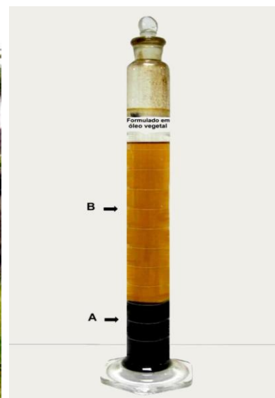
Figura 3. Conídios de M. anisopliae var. acridum (A) em óleo de soja(B), depositados no fundo do recipiente.
