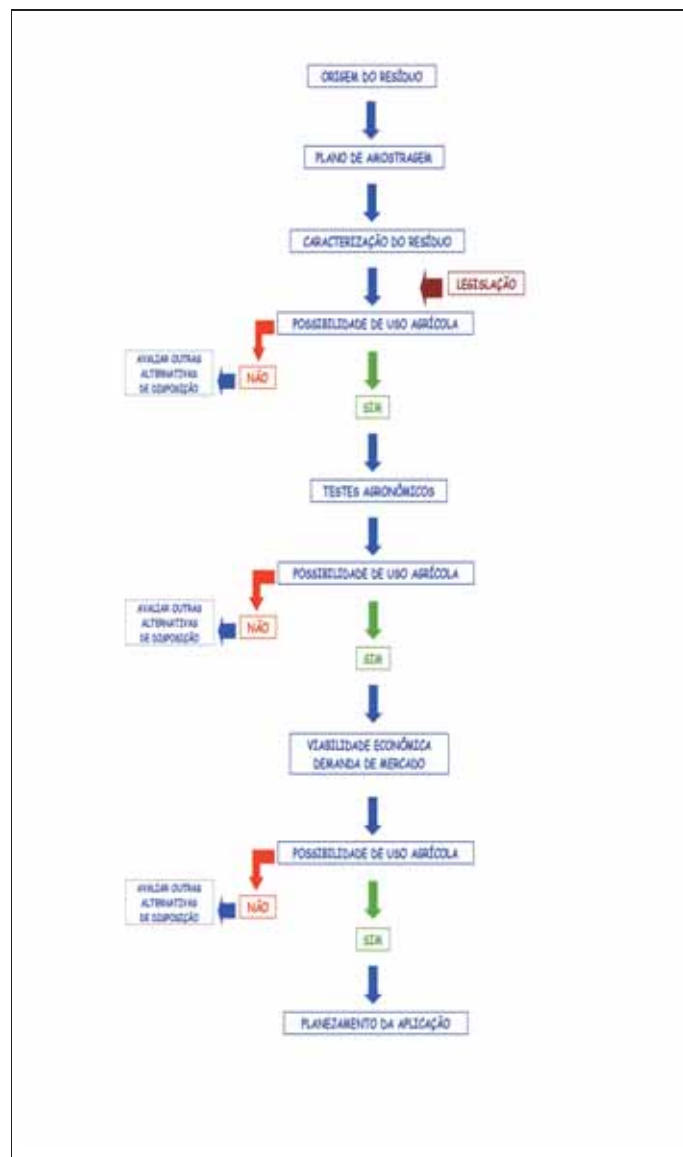
Fig. 1. Fluxograma da avaliação da viabilidade de disposição de um resíduo em solo agrícola (Adaptado de Glória, 1992 e Pires; Mattiazzi, 2005).
