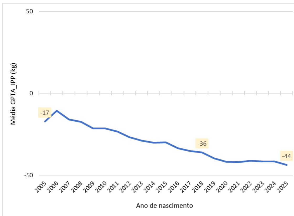
Figura 2. Tendência genética da idade ao primeiro parto (dias) por ano de nascimento.
