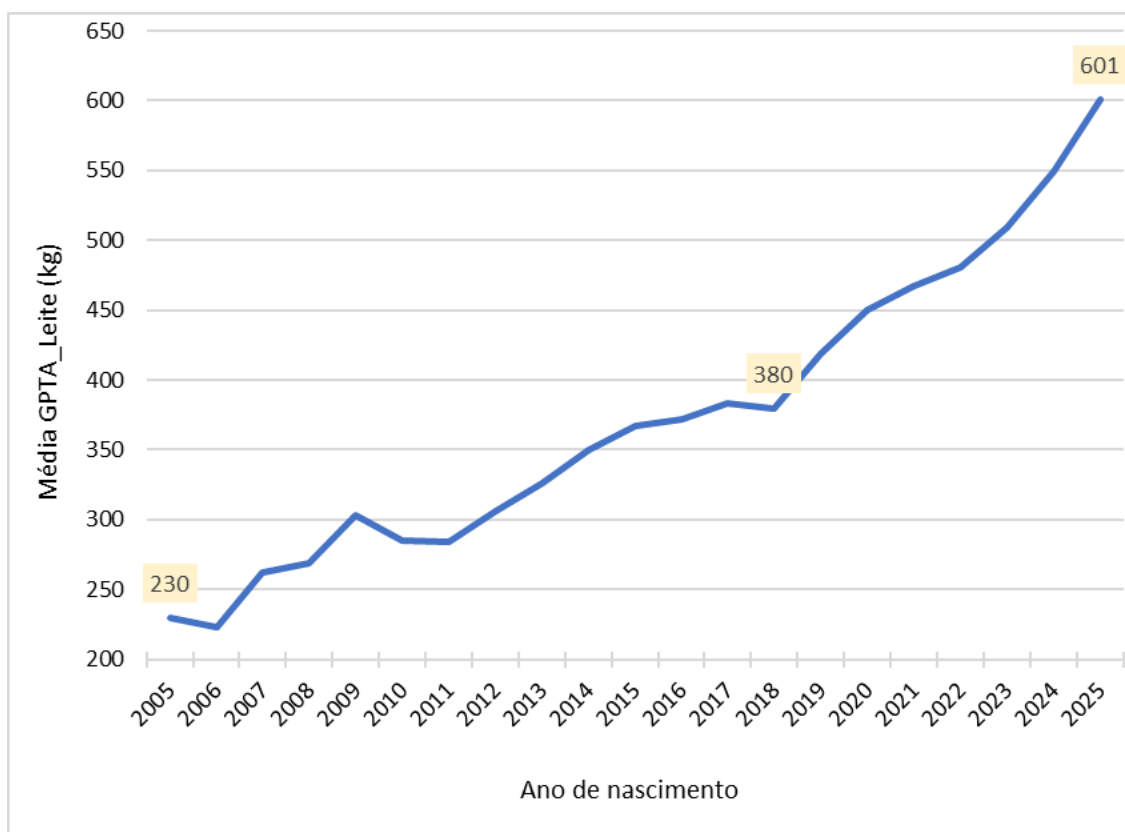
Figura 1. Tendência genética da produção de leite em até 305 dias (kg) por ano de nascimento.
