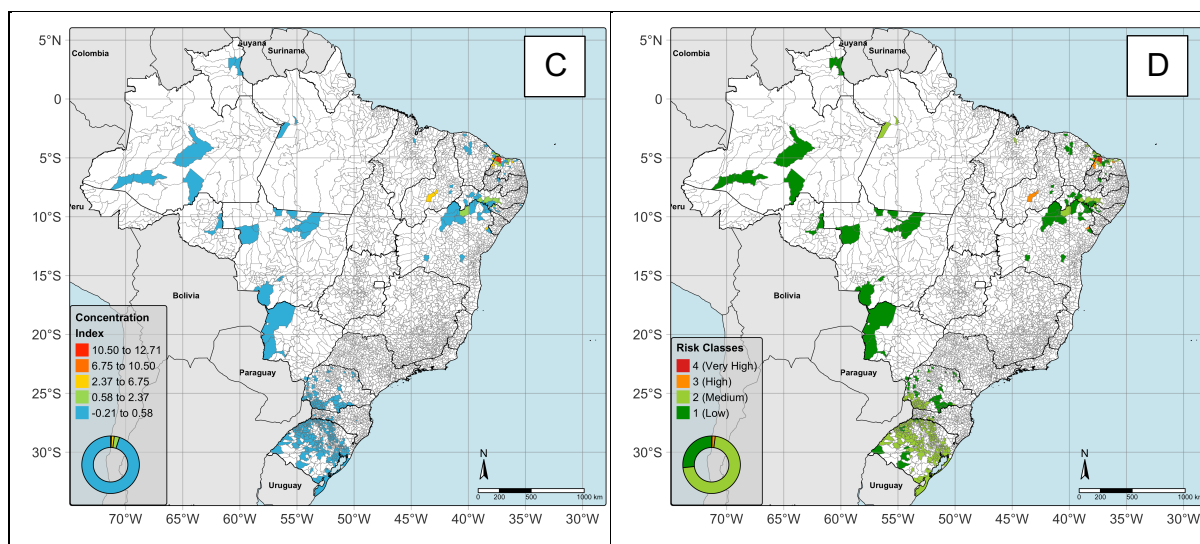
Figura 2. Modelo Maxent de probabilidade de ocorrência de Bactrocera dorsalis para o Brasil (A) e moda da probabilidade para os municípios do Brasil (B); especialização produtiva de melão pelos municípios brasileiros (C); risco econômico de B. dorsalis para produção de melão no Brasil (D).
