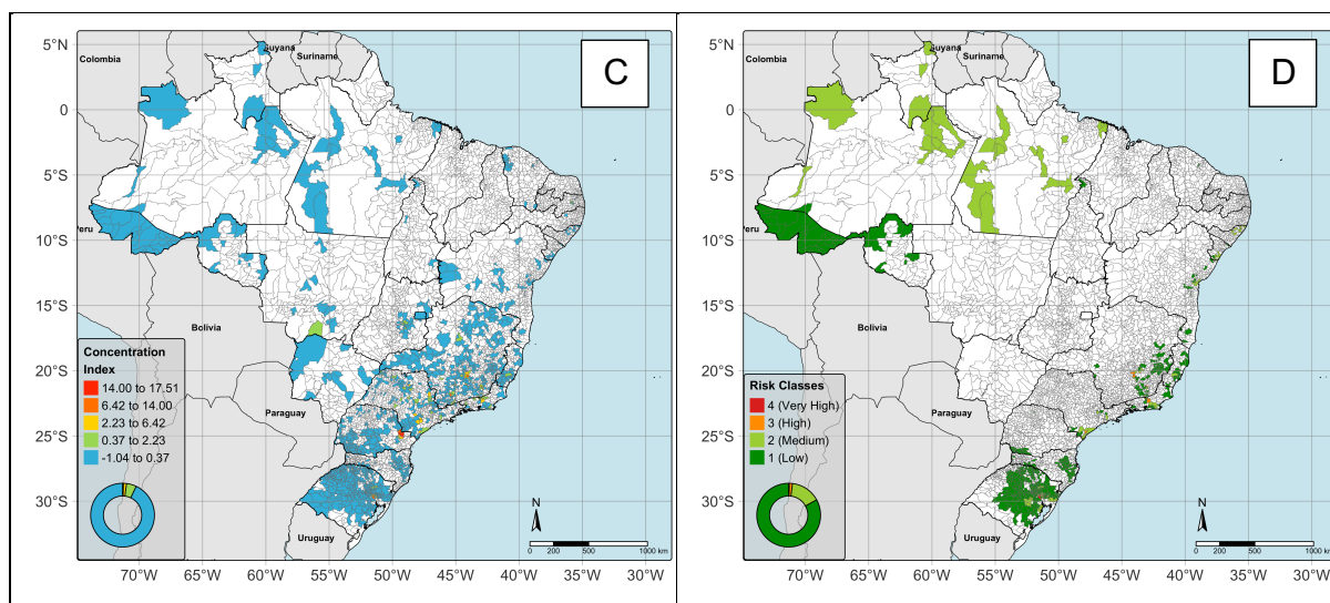
Figura 2. Modelo Maxent de probabilidade de ocorrência de Bactrocera carambolae para o Brasil (A) e moda da probabilidade para os municípios do Brasil (B); especialização produtiva de tangerina pelos municípios brasileiros (C); risco econômico de B. carambolae para produção de tangerina no Brasil (D).
