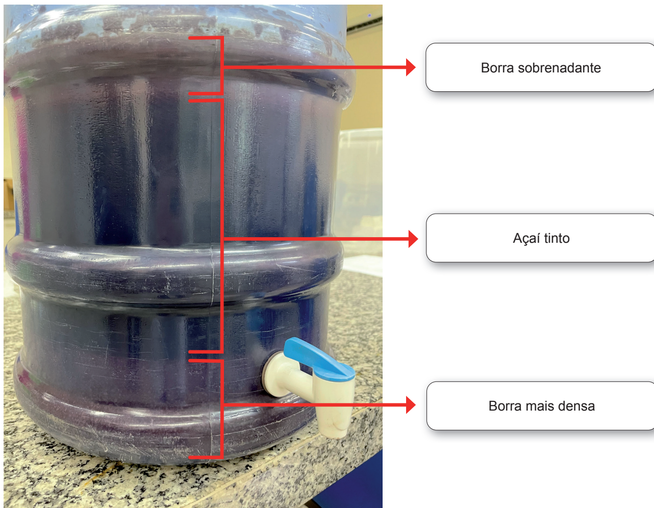
Figura 11. Fermentado bruto e as borras formadas após 23 dias de fermentação.
