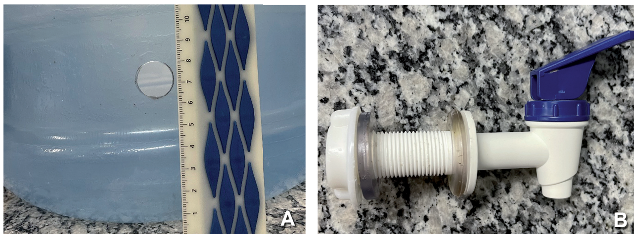
Figura 2. Altura e tamanho do furo no garrafão de água para instalação da torneira plástica de bebedouro (A); torneira plástica (B).
