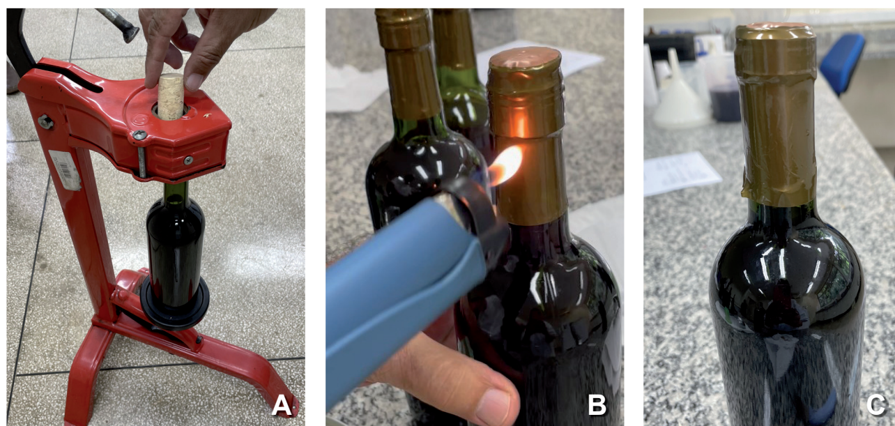
Figura 14. Processo de fechamento da garrafa com rolha de cortiça por meio de arrolhador manual (A); selagem manual com fechamento por calor (B); bebida envasada, fechada e lacrada (C).
