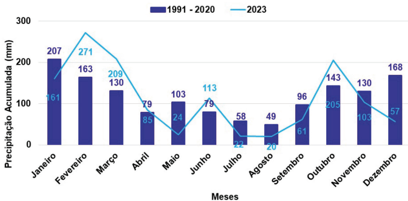
Figura 1. Precipitação pluviométrica mensal (mm) no ano de 2023 em comparação com os valores médios para o período entre 1991 e 2020. Embrapa Soja. Londrina, PR.
