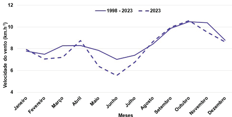
Figura 8. Velocidade do vento média mensal (km/h) no ano de 2023 em comparação ao período entre 1998 e 2023, Embrapa Soja. Londrina, PR.
