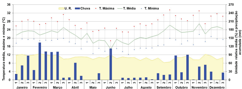
Figura 6. Valores médios de temperaturas do ar máxima, média e mínima (°C), umidade relativa (U.R.) média (%) e precipitação pluviométrica total (mm) em períodos de dez dias no ano de 2023. Embrapa Soja. Londrina, PR.
