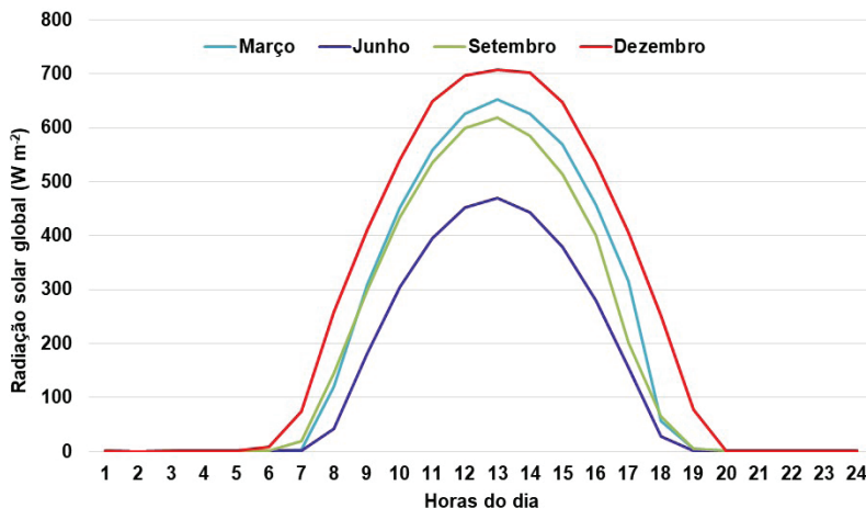
Figura 10. Radiação solar global diária ( W/m^2 ), nos dias 21 de março, 20 de junho, 26 de setembro e 20 de dezembro do ano de 2023, Embrapa Soja, Londrina, PR.
