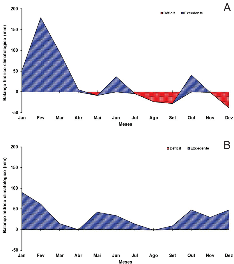
Figura 12. Valores excedentes e déficits mensais para o ano de 2023 (A) e para todo o período de coleta de dados da normal climatológica (1991 a 2020) (B), obtidos pelo balanço hídrico sequencial mensal conforme método descrito por Thornthwaite e Mather (1955), com Capacidade de Água Disponível no Solo - CAD de 75 mm, Embrapa Soja. Londrina, PR.
