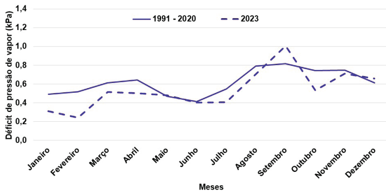
Figura 7. Déficit de pressão de vapor (kPa) no ano de 2023 em comparação ao período entre 1991 e 2020, Embrapa Soja. Londrina, PR.
