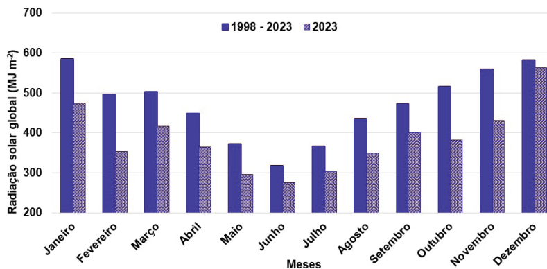
Figura 9. Radiação solar global acumulada mensalmente ( \text{MJ/m}^2 ) no ano de 2023 em comparação ao período entre 1998 e 2023, Embrapa Soja. Londrina, PR.
