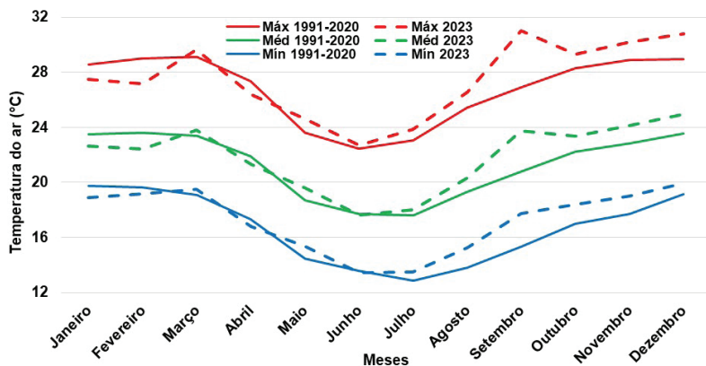
Figura 3. Temperaturas médias das máximas, médias e mínimas (°C) no ano de 2023 em comparação aos valores médios para o período entre 1991 e 2020. Embrapa Soja. Londrina, PR.
