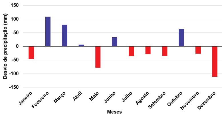
Figura 2. Desvios da precipitação pluviométrica mensal (mm) no ano de 2023 em comparação com os valores médios para o período entre 1991 e 2020. Embrapa Soja. Londrina, PR.
