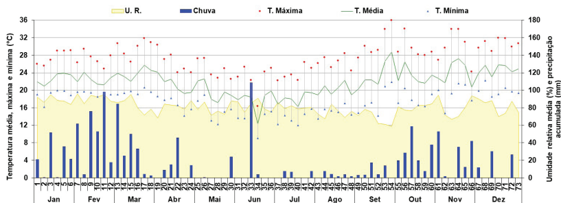
Figura 5. Valores médios de temperaturas do ar máxima, média e mínima (°C), umidade relativa (U.R.) média (%) e precipitação pluviométrica total (mm) em períodos de cinco dias no ano de 2023. Embrapa Soja. Londrina, PR.
