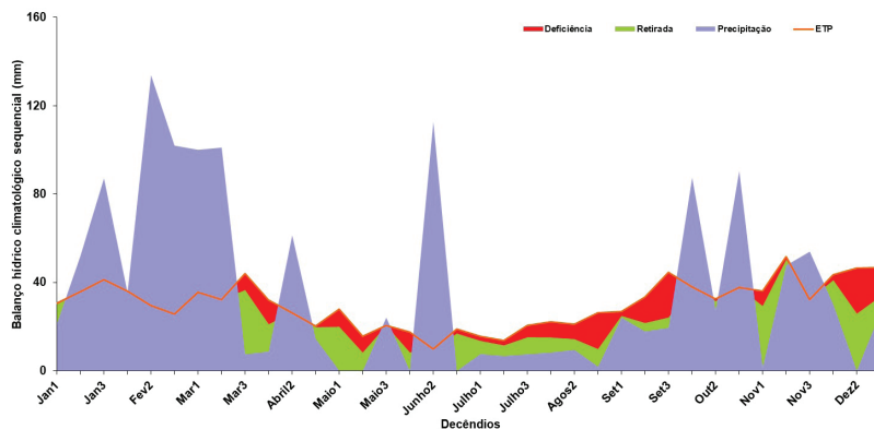
Figura 11. Balanço hídrico sequencial decenal conforme método descrito por Thornthwaite e Mather (1955), com Capacidade de Água Disponível no Solo - CAD de 75 mm e variáveis medidas no ano de 2023, Embrapa Soja. Londrina, PR.
