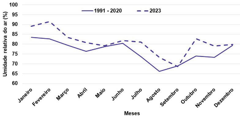
Figura 4. Umidade relativa mensal média (%) no ano de 2023 em comparação aos valores médios para o período entre 1991 e 2020. Embrapa Soja. Londrina, PR.
