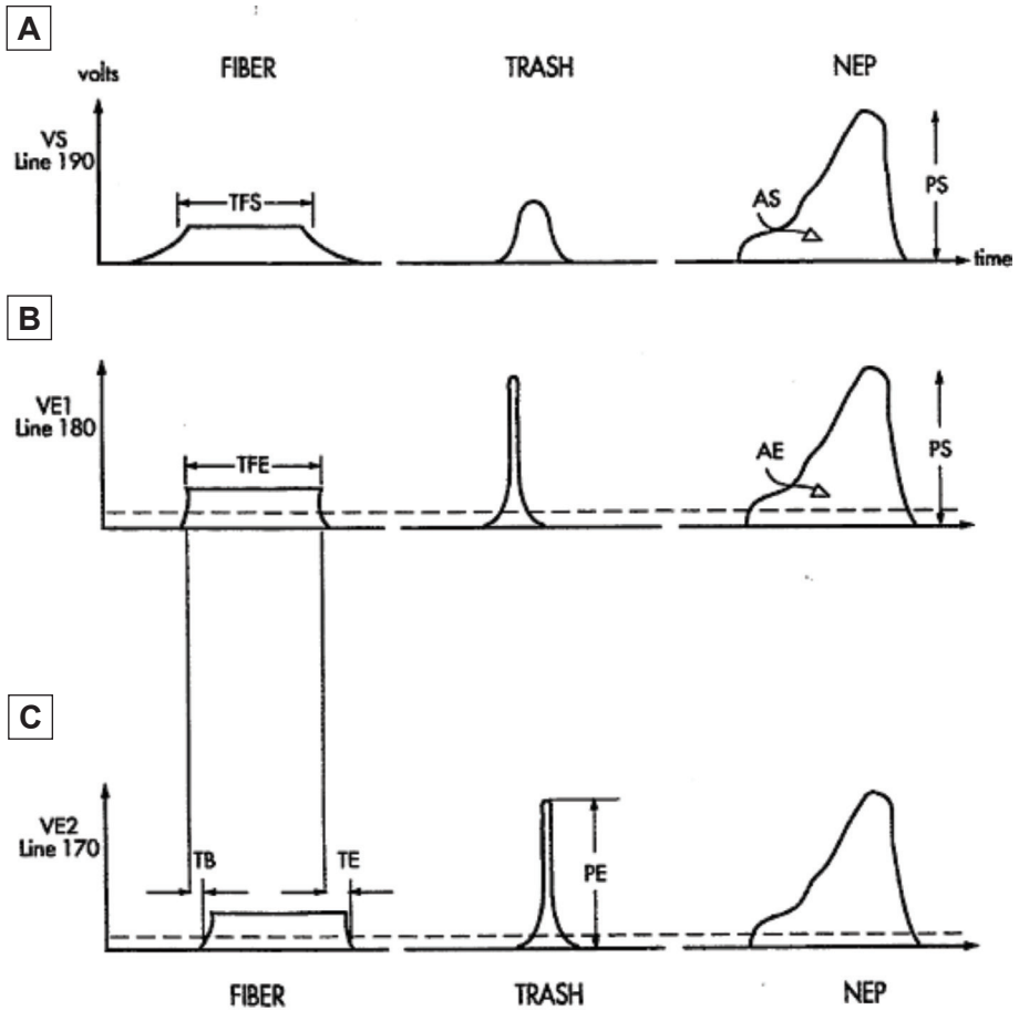
Figura 7. Exemplos de características medidas no sensor eletro-óptico do AFIS. Uma árvore de decisão é usada, baseada em limites estabelecidos, para classificar cada componente como fibra, trash ou nep.
