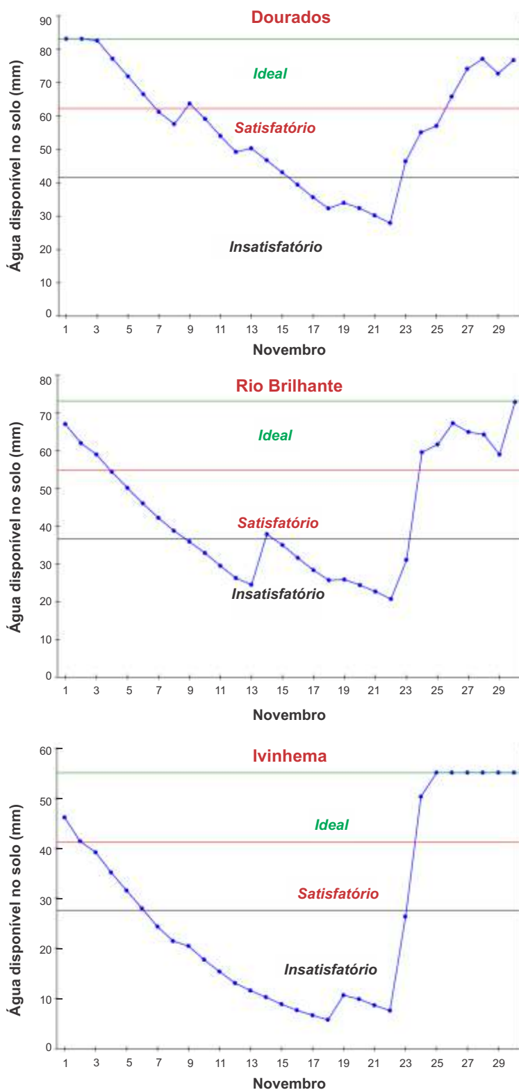
Figura 1. Balanco hídrico em Dourados, Rio Brillhante e Ivinhema, MS, em novembro de 2023.
