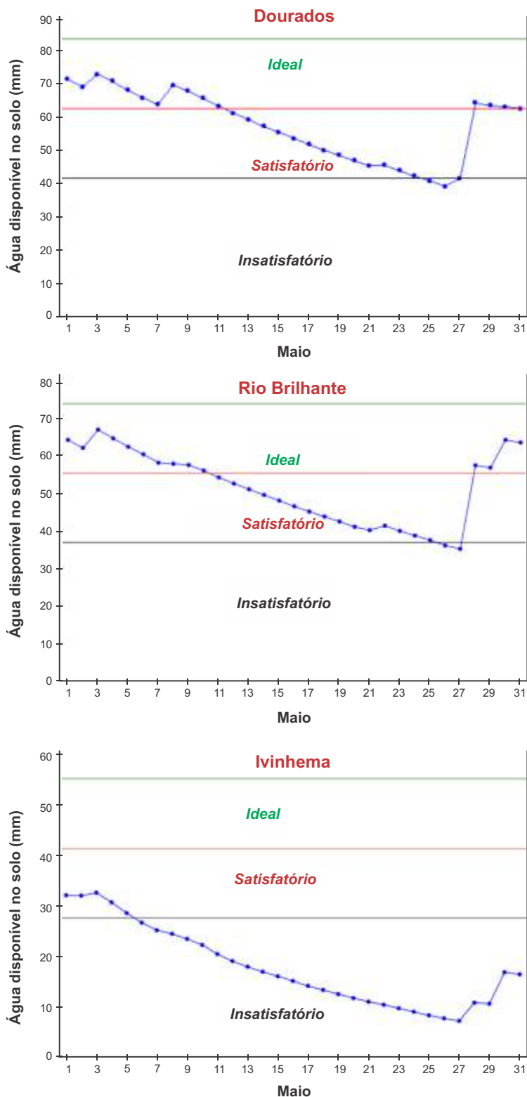
Figura 1. Balanço hídrico em Dourados, Rio Brillhante e Ivinhema, MS, em maio de 2023.
