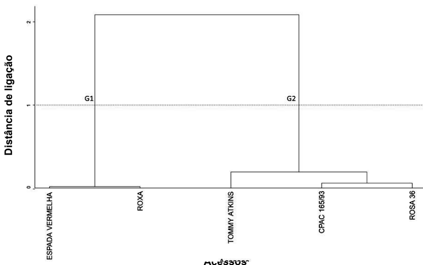
Figura 5. Dendrograma baseado na distância de Mahalanobis e método de agrupamento UPGMA de cinco genótipos de manga a partir da avaliação da severidade da antracnose em laboratório.
