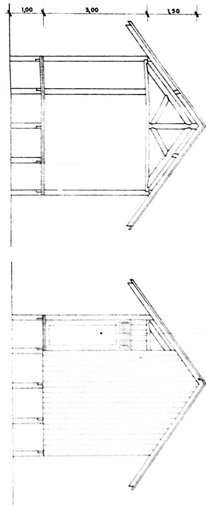
CORTE B-B' Esc 1 50
