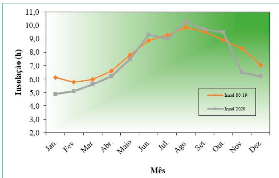
Figura 6. Valores médios mensais da insolação referentes a 2020 e ao período de 1980 a 2019. Teresina, PI.
