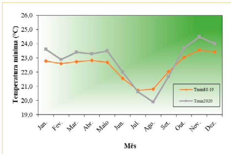
Figura 2. Valores médios mensais da temperatura mínima do ar referentes a 2020 e ao período de 1980 a 2019. Teresina, PI.
