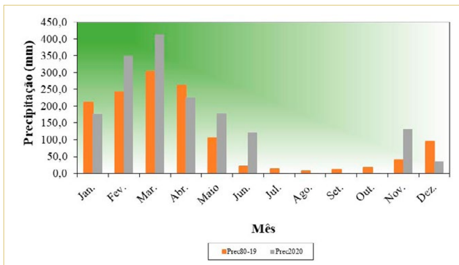
Figura 8. Totais mensais da precipitação pluviométrica referentes a 2020 e valores médios dos totais mensais da precipitação pluviométrica referentes ao período de 1980 a 2019. Teresina, PI.
