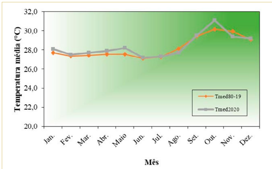
Figura 3. Valores médios mensais da temperatura média do ar referentes a 2020 e ao período de 1980 a 2019. Teresina, PI.
