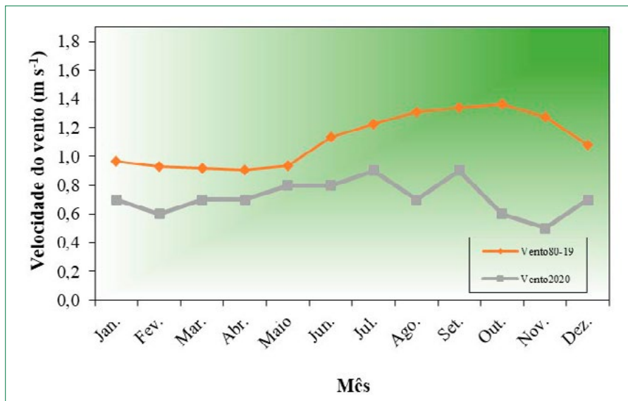
Figura 5. Valores médios mensais da velocidade do vento referentes a 2020 e ao período de 1980 a 2019. Teresina, PI.
