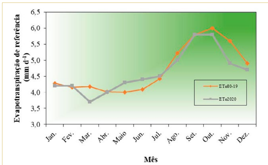
Figura 7. Valores médios mensais da evapotranspiração de referência (ETo) pelo método de Penman-Monteith referentes a 2020 e ao período de 1980 a 2019. Teresina, PI.
