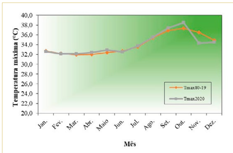
Figura 1. Valores médios mensais da temperatura máxima do ar referentes a 2020 e ao período de 1980 a 2019. Teresina, PI.
