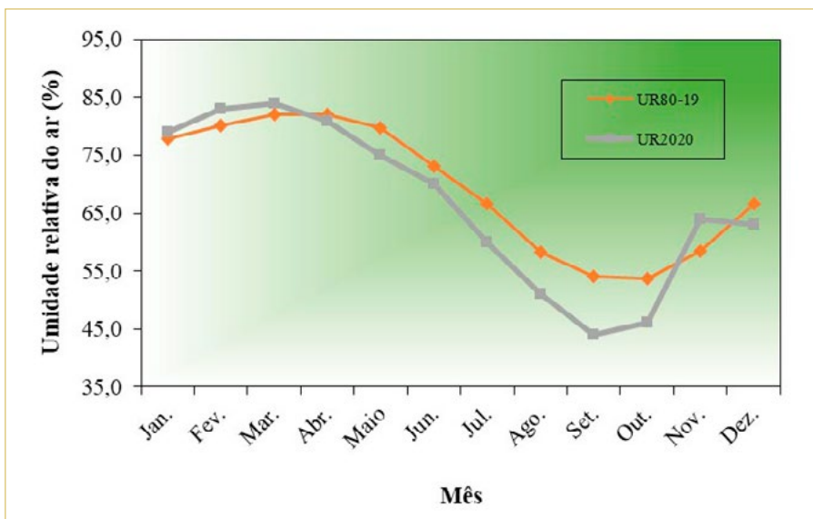
Figura 4. Valores médios mensais da umidade relativa do ar referentes a 2020 e ao período de 1980 a 2019. Teresina, PI.
