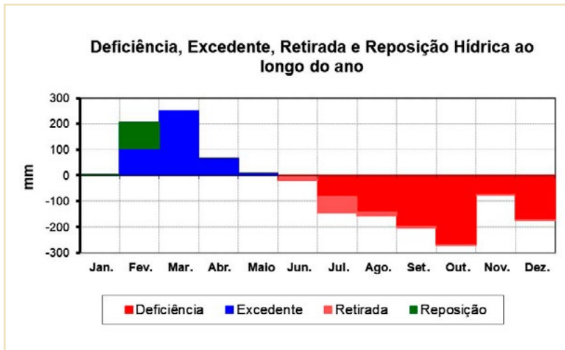
Figura 10. Extrato do balanço hídrico para o município de Teresina, PI no ano de 2020.
