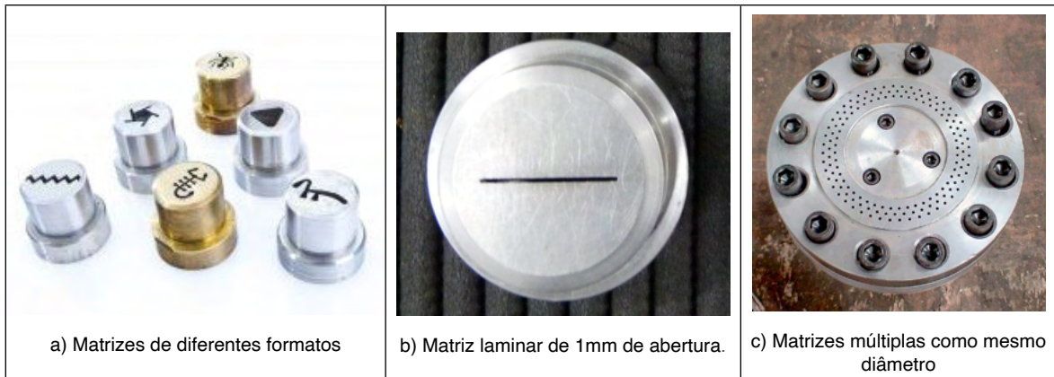
Figura 15. Diferentes tipos de matrizes a) formatos de figuras de animais e objetos; b) matriz laminar, para o produto sair como uma fita; c) matrizes múltiplas como mesmo diâmetro, típico no uso de processamento de pelets.
