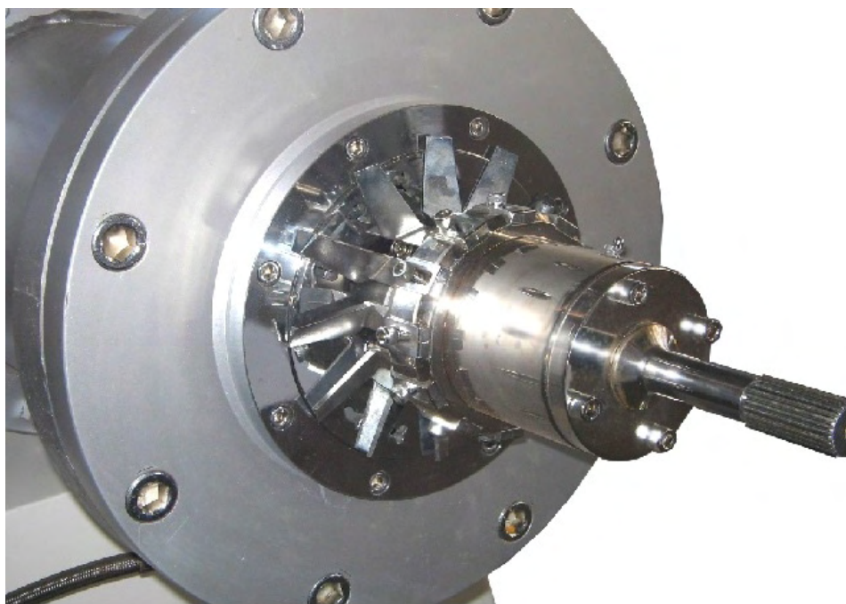
Figura 14. – Mancal de um sistema de corte, da marca Ferraz.
