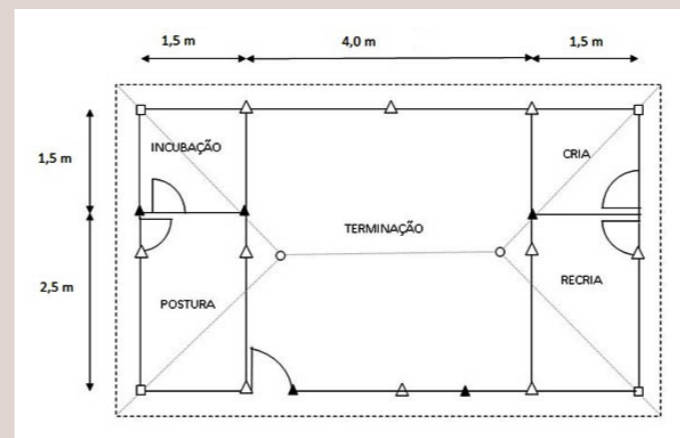
Figura 3. Planta baixa de aviário para aves caipiras de corte.
