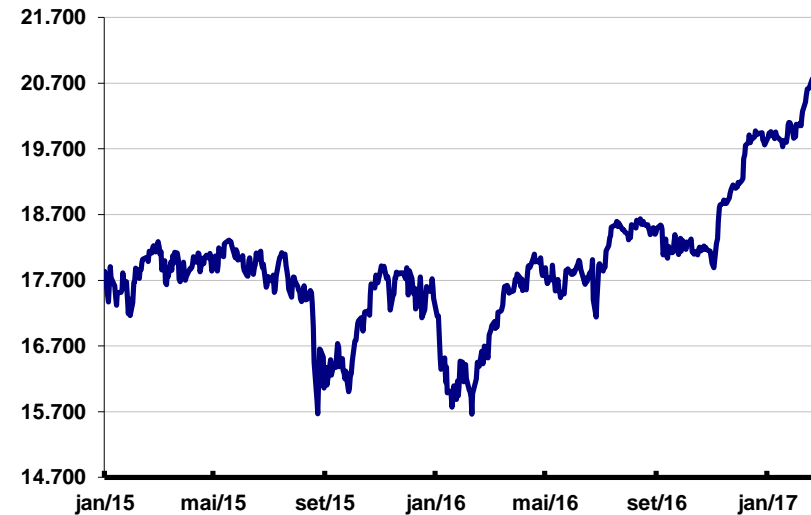
Gráfico VI.III.4 Nikkei
