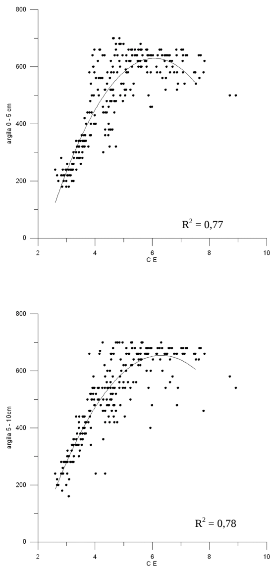
Figura 6: Correlação entre os teores de argila nas profundidades de 0 a 5 cm e 5 a 10 cm e a condutividade elétrica medida com o Veris.
