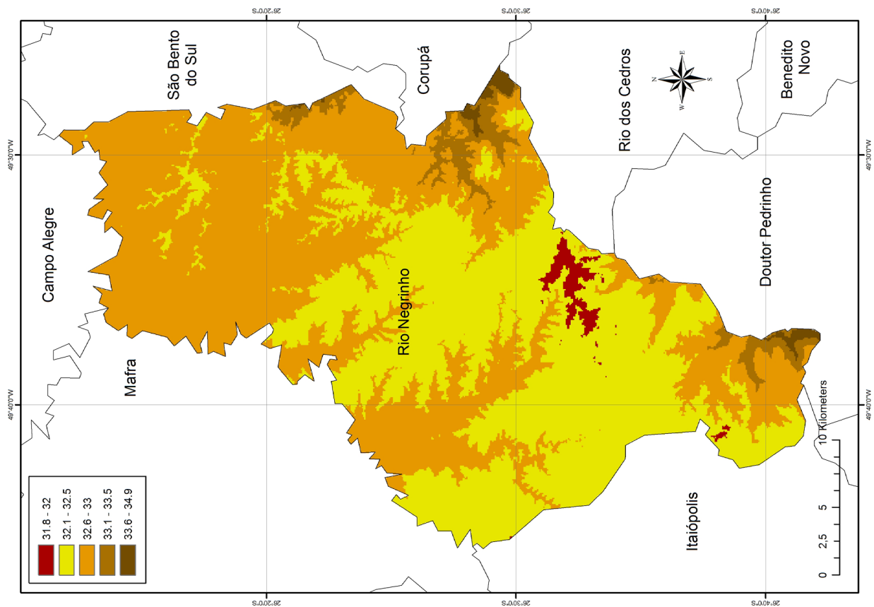
Figura 22. Mapa das médias das temperaturas máximas absolutas na primavera.
