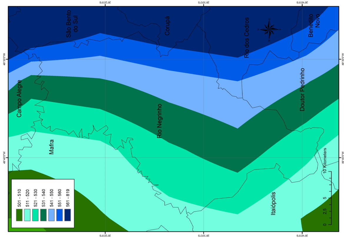
Figura 29. Mapa das médias de precipitação pluviométrica acumulada no verão.
