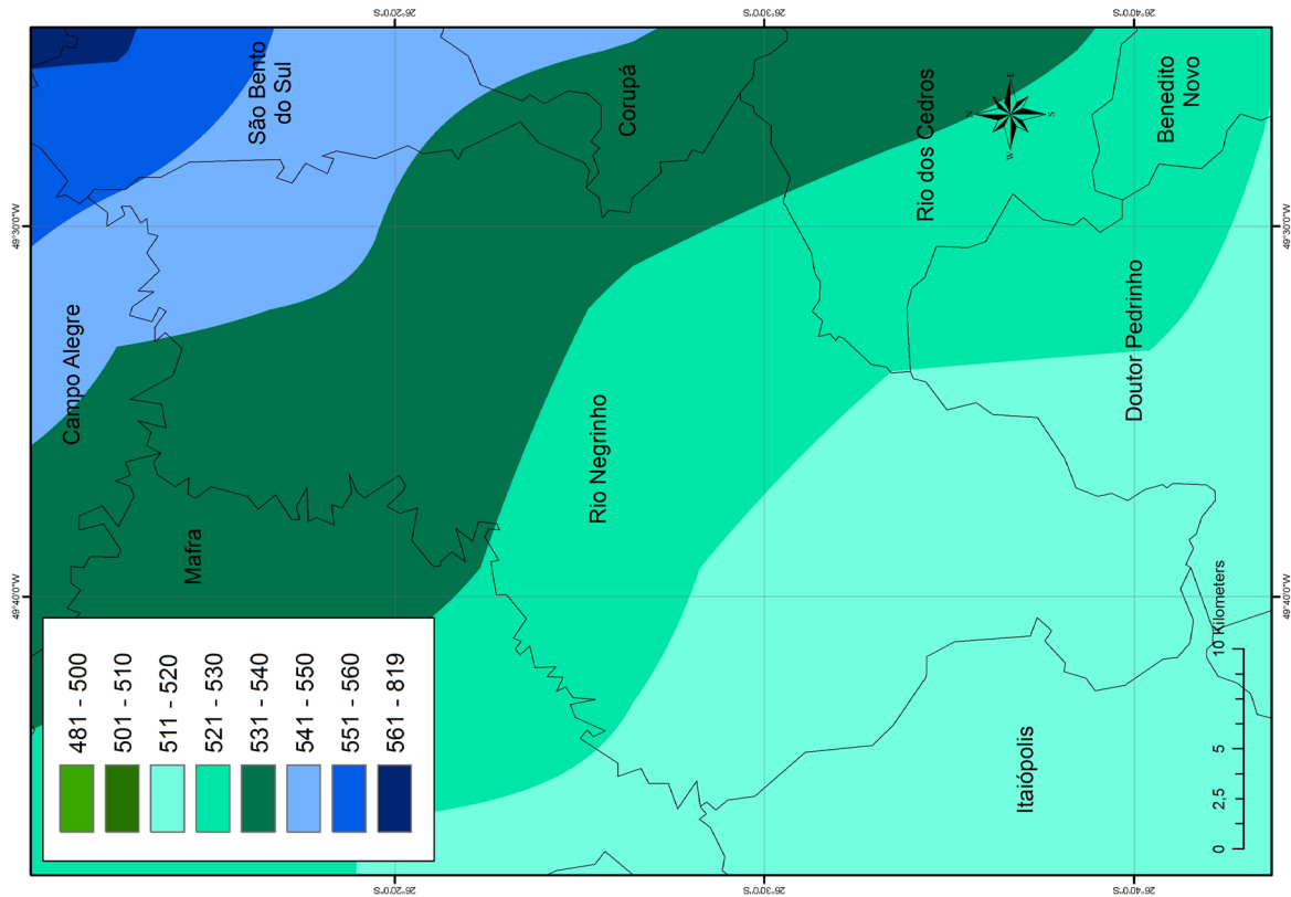
Figura 28. Mapa das médias de precipitação pluviométrica acumulada em um ano.
