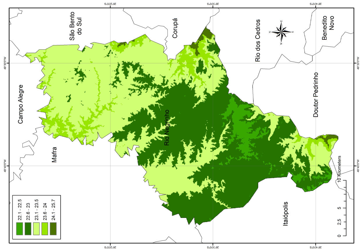
Figura 25. Mapa das médias das temperaturas máximas no outono.
