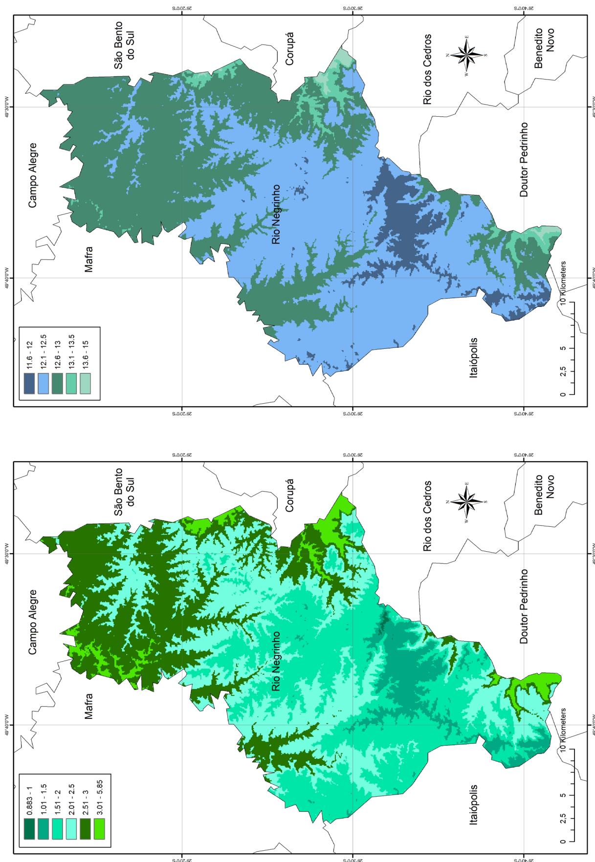
Figura 7. Mapa da média das temperaturas mínimas absolutas na primavera.
