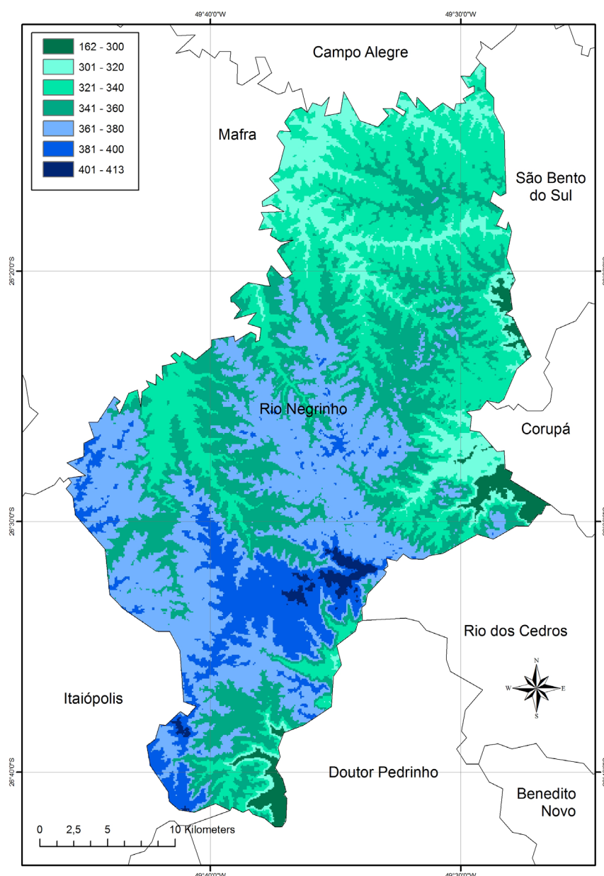
Figura 2. Mapa das horas de frio (<7,2 °C) acumuladas no outono-inverno (maio-setembro).
