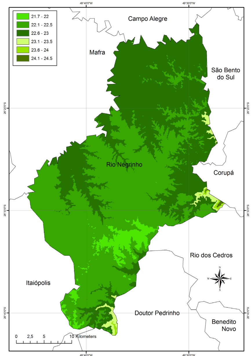
Figura 27. Mapa das médias das temperaturas máximas na primavera.
