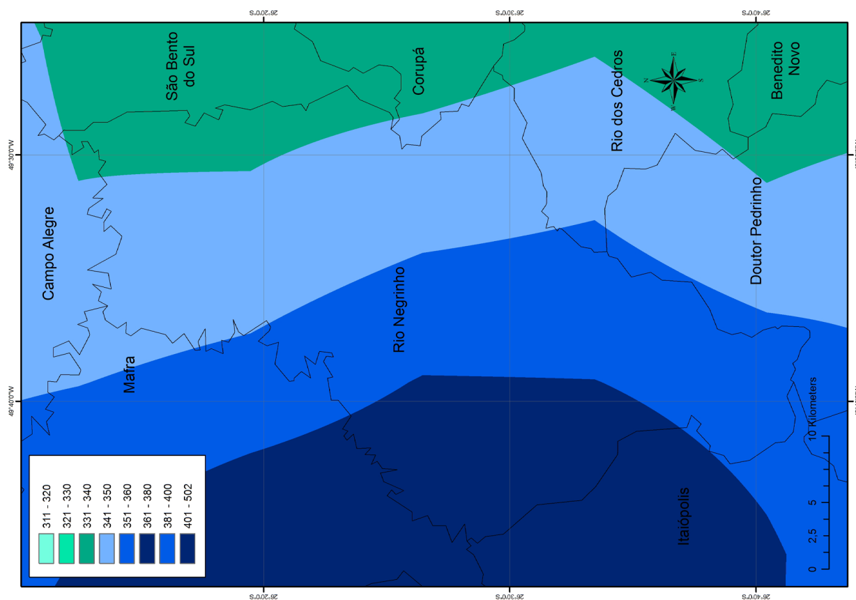
Figura 31. Mapa das médias de precipitação pluviométrica acumulada no inverno.
