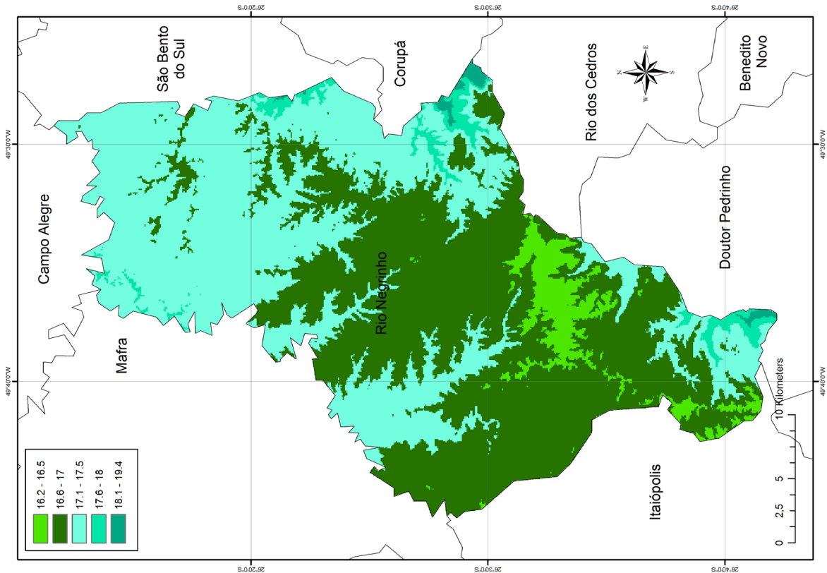
Figura 13. Mapa das temperaturas médias no ano.
