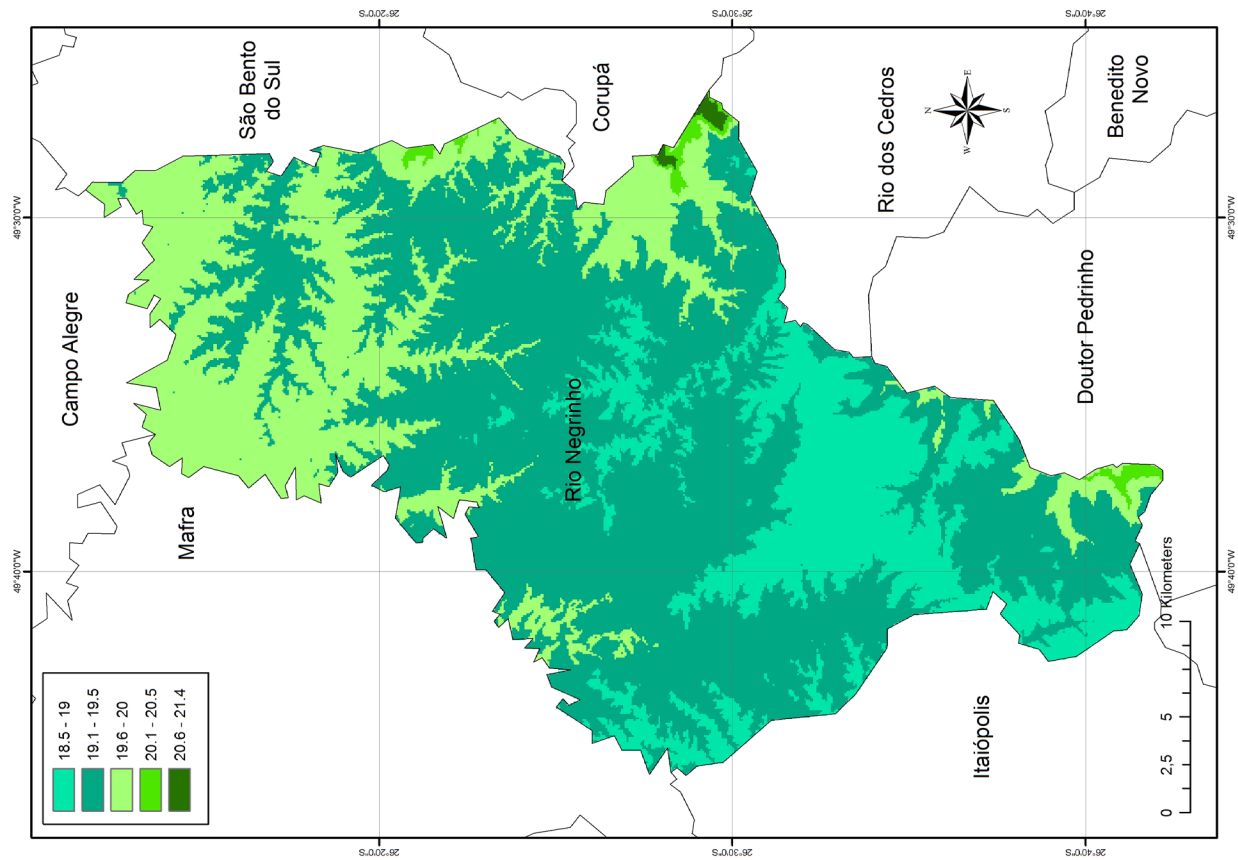
Figura 26. Mapa das médias das temperaturas máximas no inverno.
