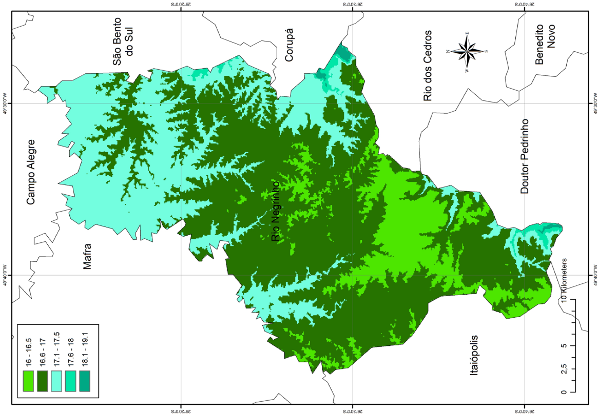
Figura 17. Mapa das temperaturas médias na primavera.
