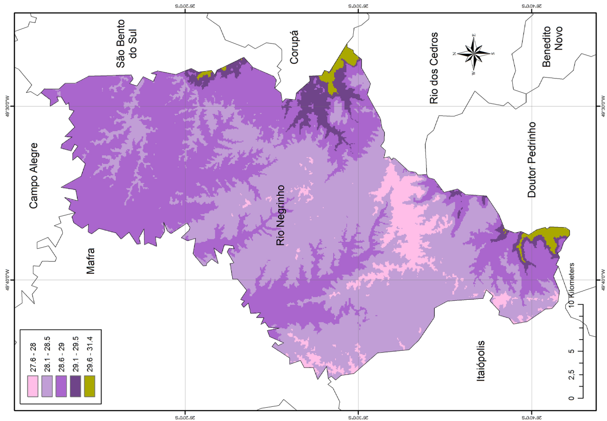
Figura 21. Mapa das médias das temperaturas máximas absolutas no inverno.
