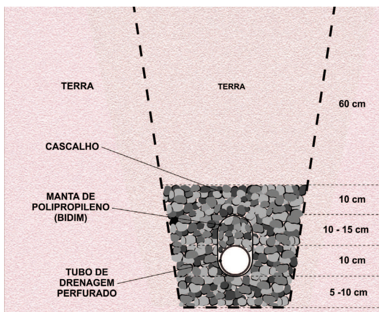
Figura 4. Sistema de drenagem utilizando brita, tubos corrugados perfurados em polietileno de alta densidade (PEAD) e manta de polipropileno.
