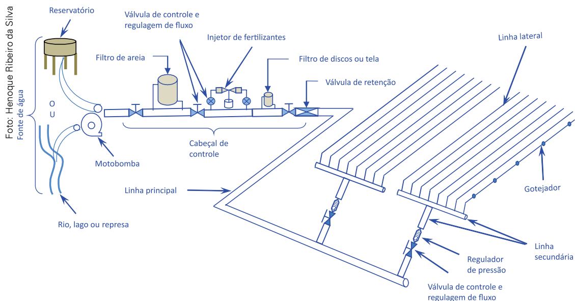
Figura 26. Esquema básico de instalação de um sistema de rega por gota-a-gota não automatizado.
