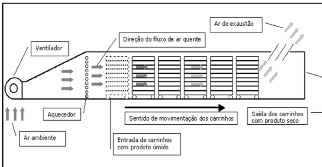
Figura 82. Esquema do secador tipo túnel concorrente.
