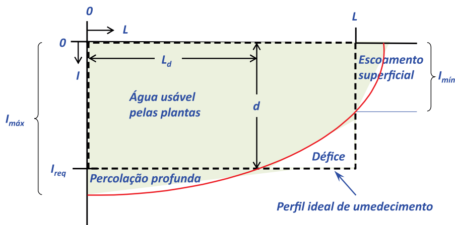
Figura 38. Perfil de humedecimento do solo ao longo do sulco durante o evento da irrigação.
