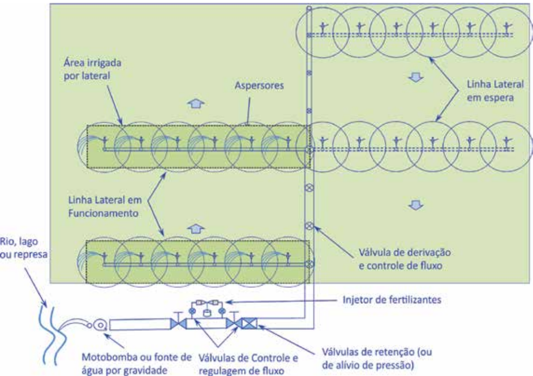
Figura 25. Esquema básico de montagem e funcionamento de um sistema de rega por aspersão convencional portátil com duas linhas laterais em funcionamento.
