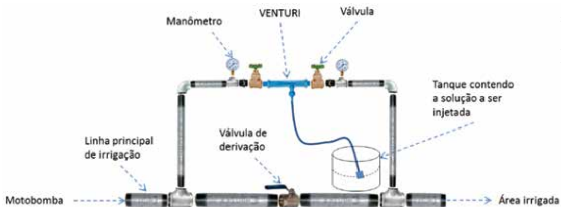
Figura 36. “Layout” de montagem do dispositivo venturi para injeção de soluções fertilizantes em sistemas de irrigação pressurizados.
