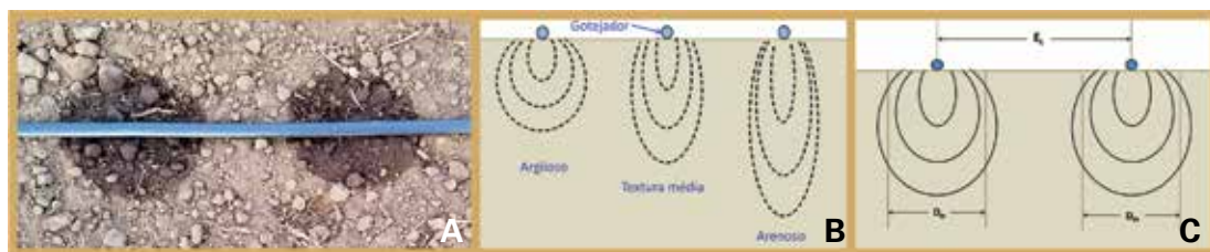
Figura 28. (A) Foto da área molhada e formação da faixa molhada em condições de campo. (B) Formato do bolbo molhado em função da textura do solo. (C) Cálculo estimativo do bolbo molhado e espaçamento entre linhas laterais.
