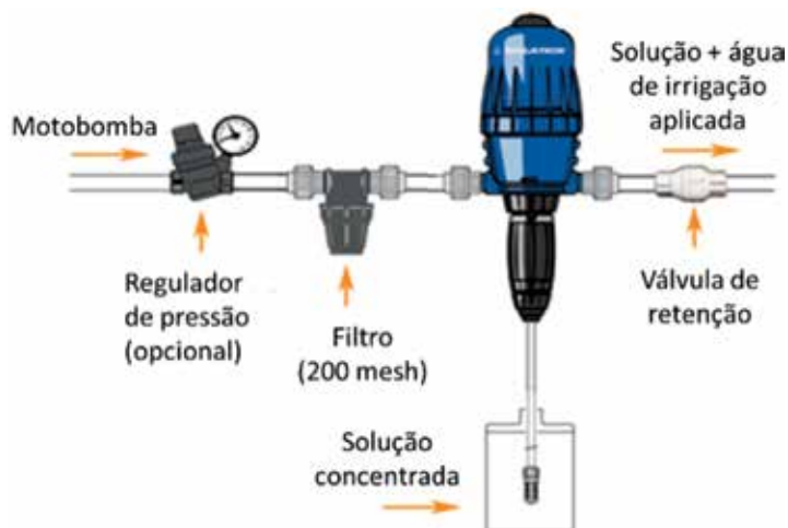
Figura 35. Exemplo de montagem de uma bomba dosadora.
