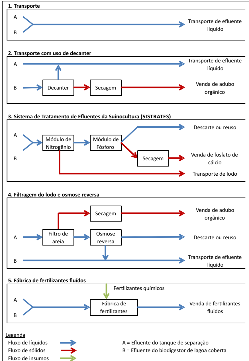
Figura 3. Alternativas tecnológicas consideradas para o correto manejo e disposição final dos efluentes de uma usina central de biogás em Tupandi, RS
