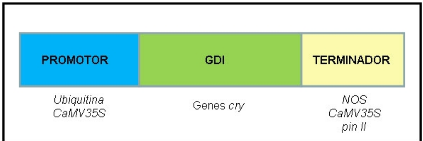
Figura 07: Principais regiões componentes de um gene. Ubiquitina e CaMV35S: exemplos de promotores utilizados para direcionar a expressão dos genes cry; NOS, CaMV35S e pin II: exemplos de regiões terminadoras utilizadas para finalizar a transcrição dos genes cry
