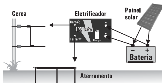
Fig. 2. Esquema de ligação do Eletrificador de 12 Volts com painel solar e bateria.
